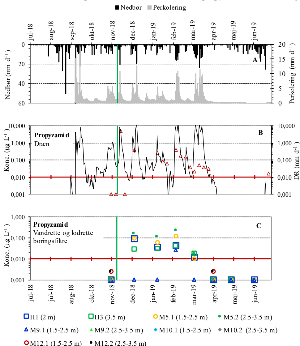
Figur B2.1. Monitoringsresultater for propyzamid-udvaskningstesten i Silstrup 2018-2019 : (A) målt nedbør og simuleret perkolerung i 1 meters dybde angivet i lineær skala, (B) koncentrationen af propyzamid i drænvandsprøver og drænvandsafstrømningen angivet i log-skala og (C) koncentrationen af propyzamid i grundvandsprøver udtaget fra lodrette boringsfiltre (M) og vandrette boringsfiltre (H). Boring M12 er placeret opstrøms for marken angivet i log-skala. I tilfælde af at der ikke er fundet propyzamid i vandprøven tilføjes punktet på plottet værdien 0,001 µg/L og for M12 0,0025 µg/L – altså en værdi under detektionsgrænsen på 0,01 µg/L (den røde x-akse). Den grønne lodrette streg angiver datoen for sprøjtningen med propyzamid.
