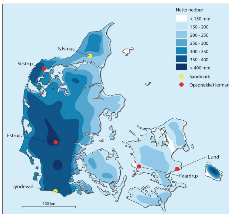
Figur 1. VAP-markernes placering i forhold til nettonedbør, der angiver andelen af nedbør, som når grundvandet. Markerne, der indgår i VAP, repræsenterer de mest udbredte danske klima- og jordtyper, hvori sandjorde og opsprækkede lerjorde indgår. (MST-rapport nr. 87-503-9581-5, 1992).
