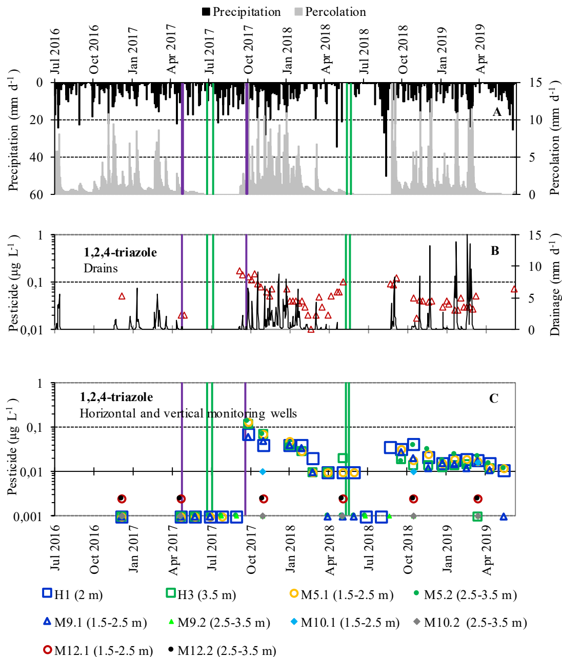
Figur B1.3. Udvalgte monitoringsresultater for 1,2,4-triazol-udvaskningstestene fra opsprækkede lermark Silstrup 2016-2019 : (A) målt nedbør og simuleret perkolering i 1 meters dybde angivet i lineær skala, (B) koncentrationen af 1,2,4-triazol i drænvandsprøver angivet i log-skala og drænvandsafstrømningen DR angivet i lineær skala og (C) koncentrationen af 1,2,4-triazol i grundvandsprøver udtaget fra lodrette boringsfiltre (M) og vandrette boringsfiltre (H) angivet i log-skala. Boring M12 er placeret opstrøms for marken. I tilfælde af at der ikke er fundet 1,2,4-triazol i vandprøven tillægges punktet på plottet værdien 0,0025 µg/L, hvis prøven er fra den opstrøms boring M12, eller gives værdien 0,001 µg/L – altså værdier under detektionsgrænsen på 0,01 µg/L (x-akse). De grønne lodrette streger angiver i tidspunktet for sprøjtningen med propiconazol to gange i 2017 og prothioconazol to gange i 2018. De lilla streger angiver anvendelsen af såsæd bejdset med tebuconazol og prothioconazol. Det skal bemærkes, at bejdsemidler anvendt på såsæd anvendt i VAP blev registreret fra 2017.
