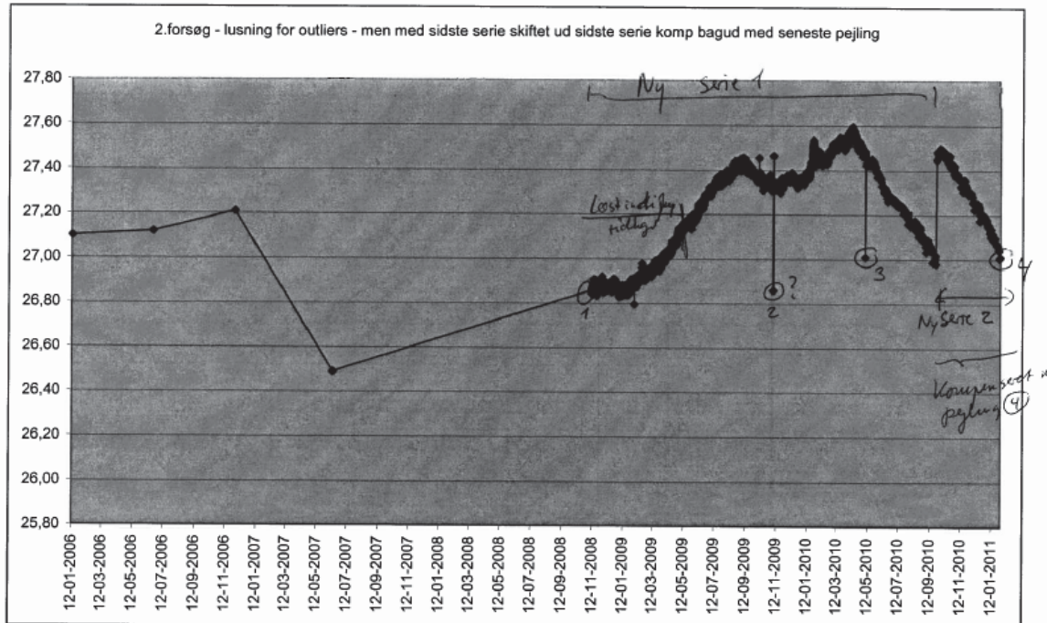
Figur 10. Oprettning af data. Denne tidsserie kasseres helt, da Diveren tilsyneladende driver flere meter og tidsserien kan ikke rettes op så de passer med de manuelle pejlinger.
