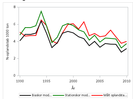
Biasregion 4
