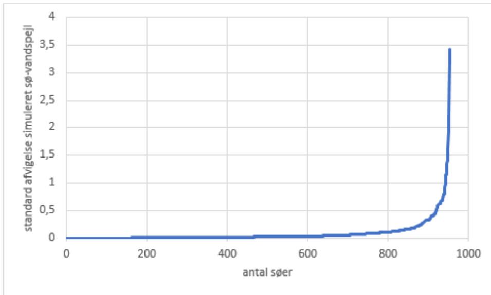
Figur 12: Beregnede variationer af afvigelser fra simuleret 'vandret' søvandspejl.
