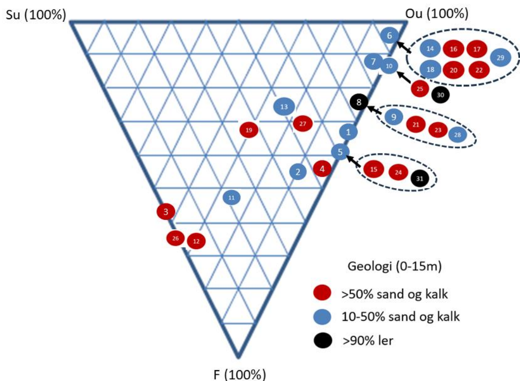
Figur 21: Ud-budgettet for 31 testsøer beregnet med DK-model2023. Sønumre er vist i legende til Figur 20.
