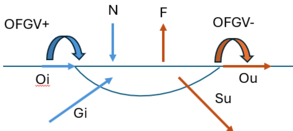
Figur 17: Vandbalancens komponenter. Modelteknisk udgør forskellen på OFGV+ og OFGV- den overfladenære grundvandstilstrømning.
