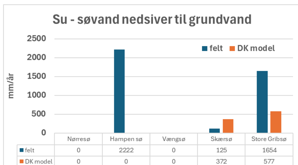
Figur 19: Udsivning af søvand til grundvandszonen kvantificeret med feltmålinger og DK-model2023.
