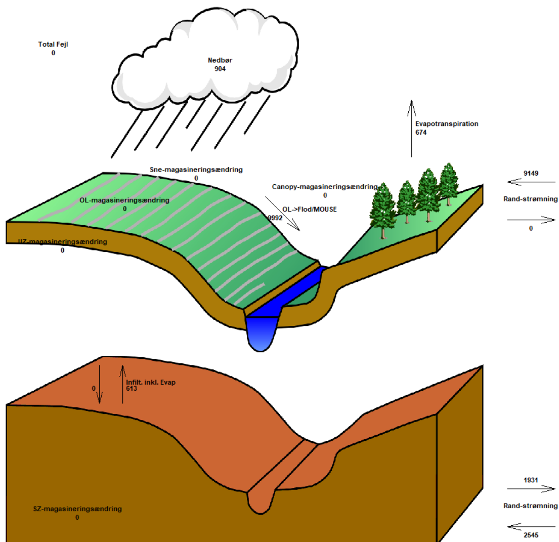
Figur 15: Vandbalance for Vængsø i mm/år som MikeSHE udtræk.
