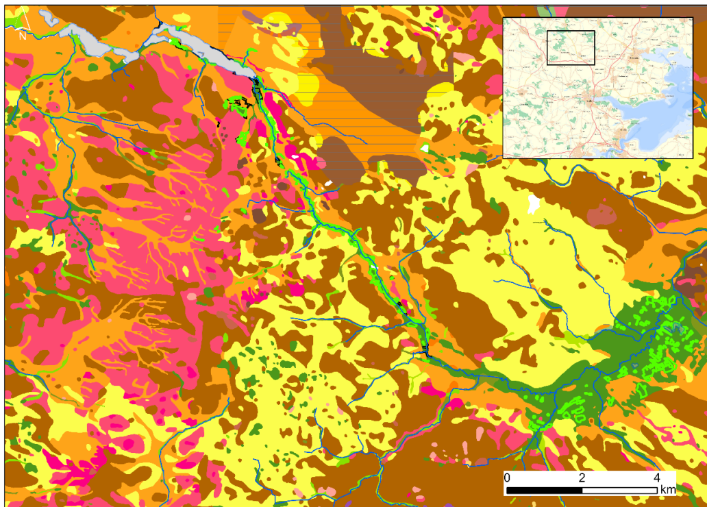
Figur 5: GATØ afgrænsninger i ådal nord for Vejle. GATØ afgrænsninger er angivet som grønne polygoner og grundvandsafhængige skov habitatområder med sorte polygoner.
