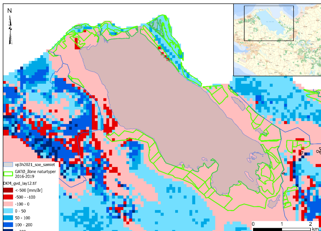
Figur 8: Grundvandsdannelse (flux) til øverste beregningslag (negative tal angiver opadrettet gradient) for GATØ beliggende ved Kalundborg
