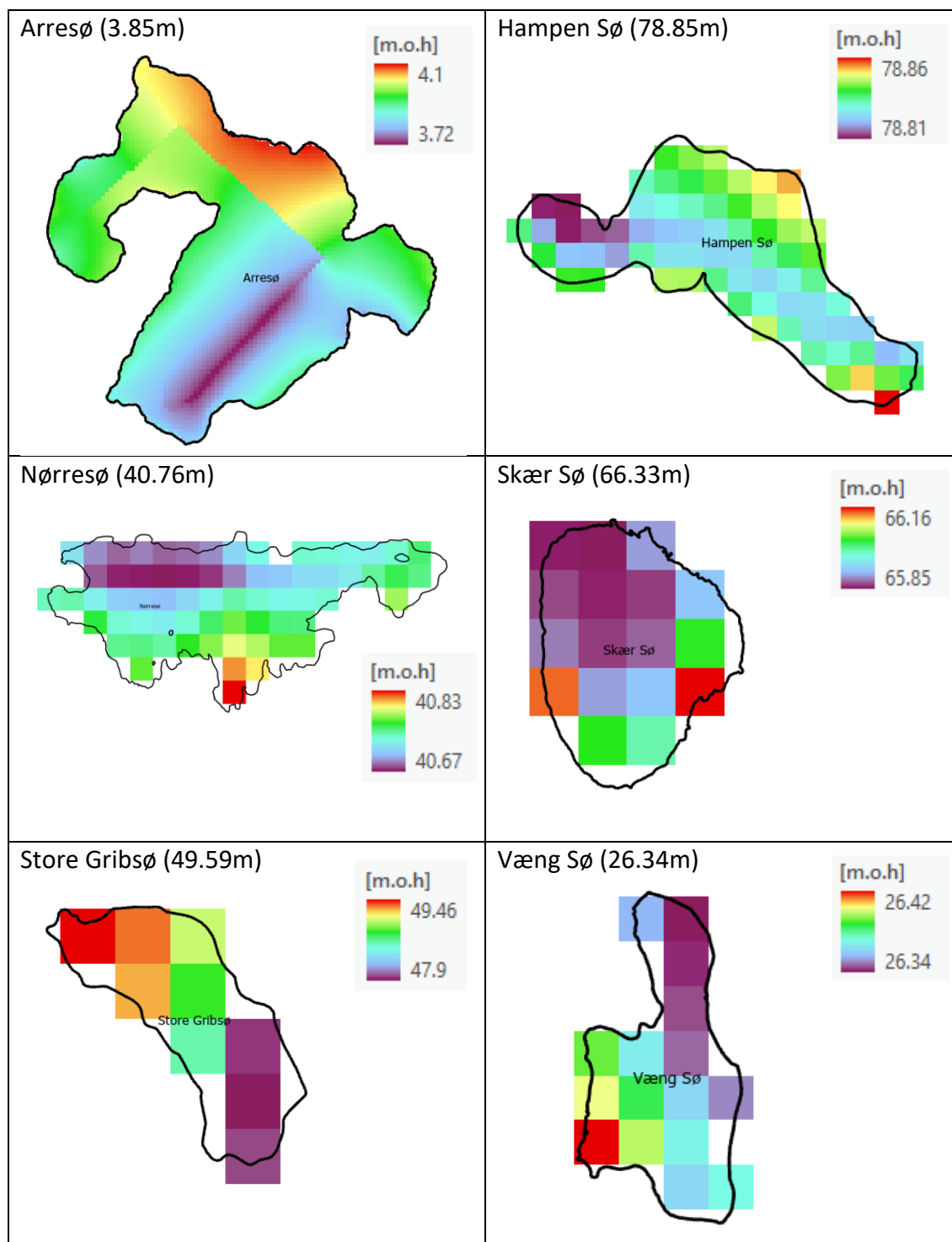
Figur 11: Simuleret vandstand i eksempel søer. Initial sø vandstandskote i parentes, simuleret vandstand som middel 2001-2018 indenfor modellens søareal. Søernes størrelse afspejles af antallet af beregningsgrids i hver sø.
