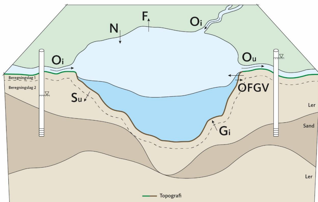
Figur 14: Konceptuel skitse af modelberegnet vandbalance med søkonceptet i DK-model2023. Forkortelser: Nedbør (N), fordampning (F), overfladisk indstrømning ( O_i ), overfladisk udstrømning ( O_u ), grundvandsindstrømning ( G_i ), udsivning af søvand til grundvand ( S_u ), overfladenær grundvandsindstrømning (OFGV).
