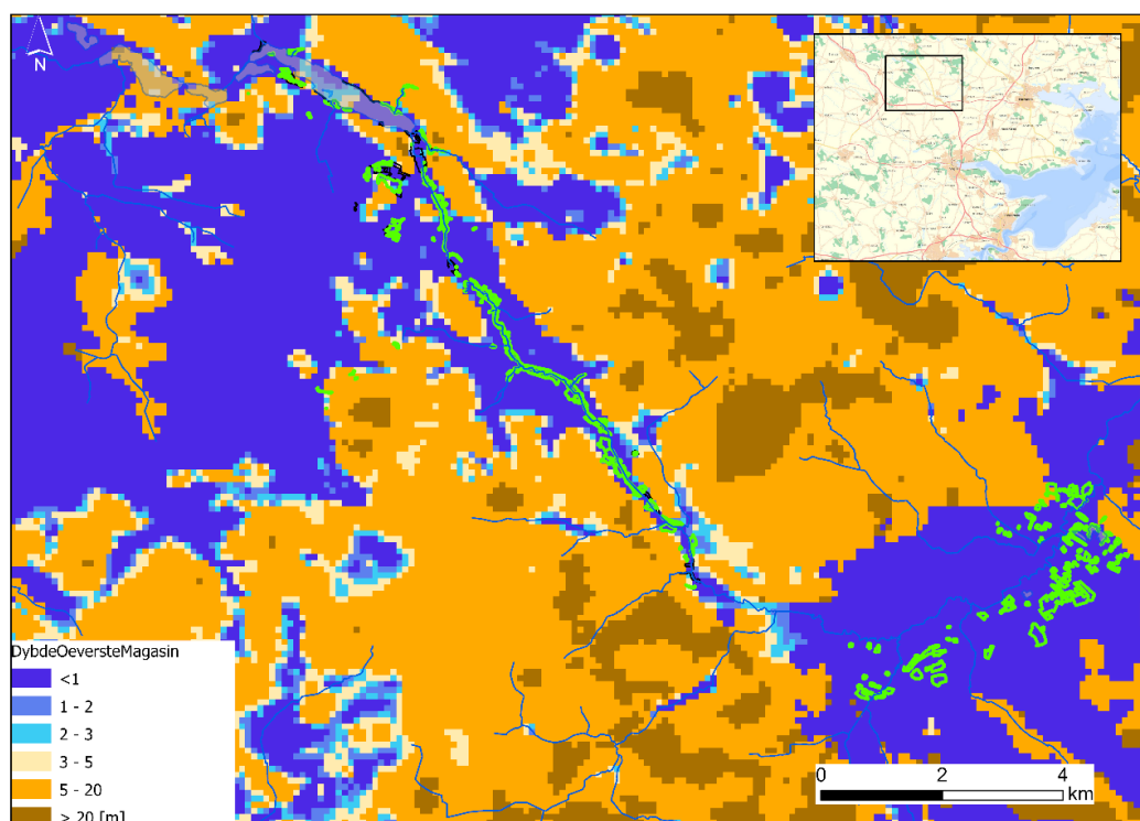
Figur 6: Dybde til øverste grundvandsforekomst og GATØ afgrænsninger i ådal nord for Vejle
