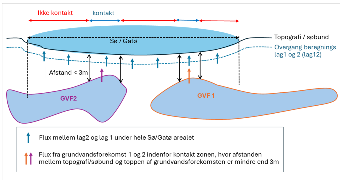
Figur 3: Tværsnit principskitse af afstandskriterie og modelsimuleret vandudveksling mellem søer og grundvandsforekomster. For det samlede sø-areal opgøres den opadrettede grundvandstilstrømning til det øverste beregningslag, mens den magasinsspecifikke opadrettede strømning kun opgøres for kontaktarealet, svarende til den del af sø-arealet hvor afstanden er mindre end 3 meter til toppen af grundvandsforekomsten og der er opadrettet strømning.
