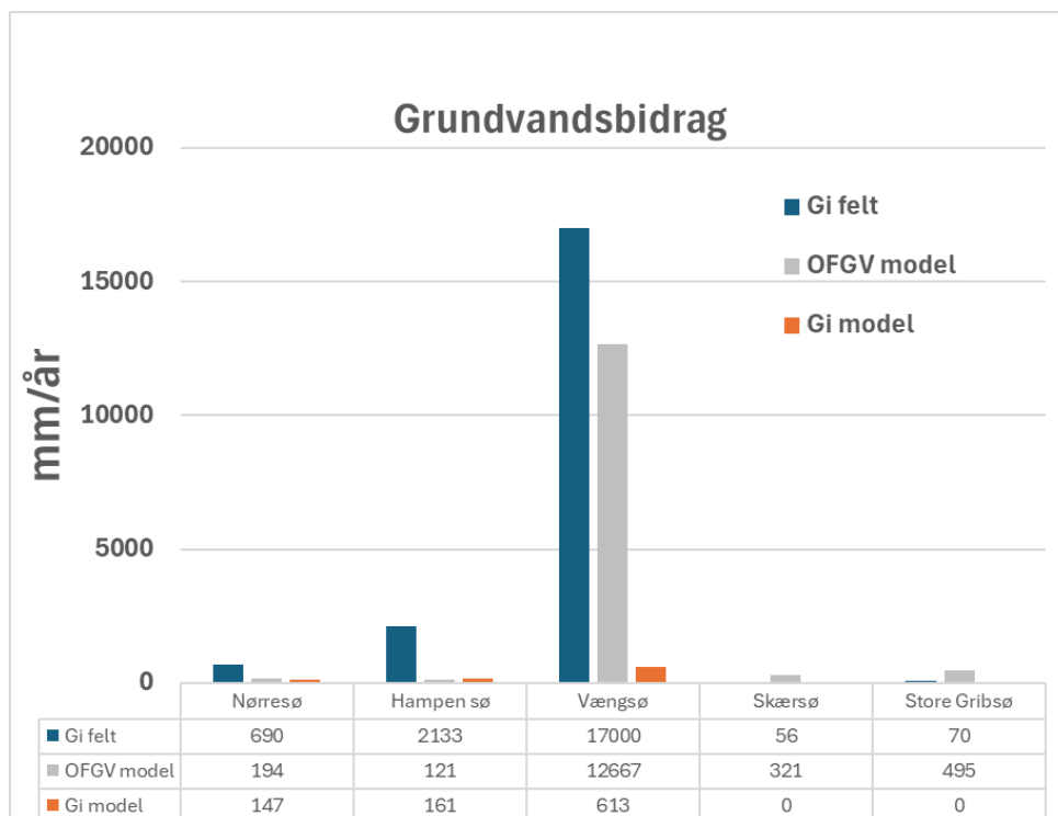
Figur 18: Grundvandsbidraget til de fem testsøer kvantificeret med feltmålinger og DK-model2023.
