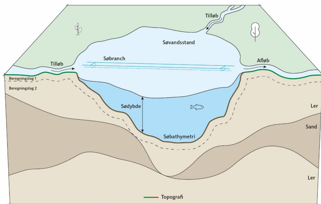
Figur 9: Justeret sø-koncept. Søbathymetrien er indbrændt i den topografiske model. Hver sø har egen vandløbsopsætning med en søbranch og op til flere vandløbstilløb. Vandspejlsdybder større end sødybden, bidrager med overfladestrømning
