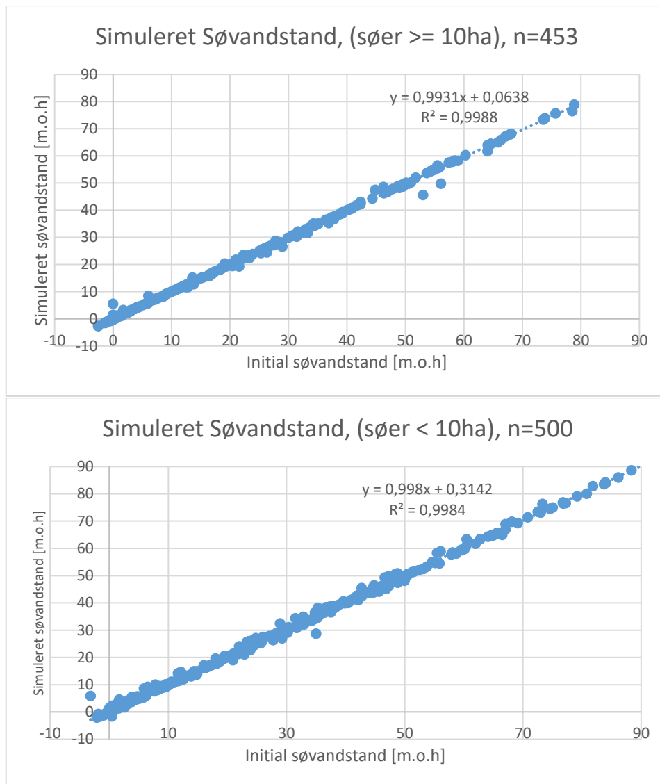
Figur 10: Simuleret søvandstand ift initial søvandstand.
