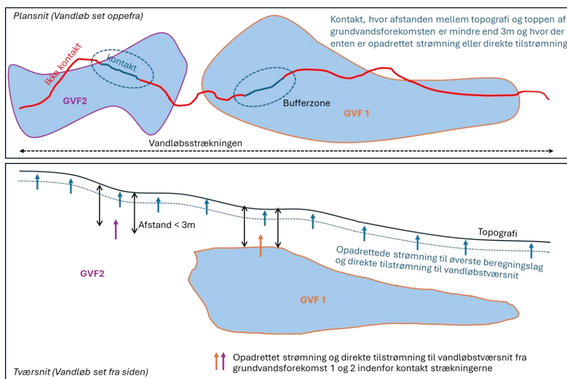
Figur 2: Principskitse for grundvandsforekomst kontaktvurdering og strømningsberegninger (flux) for vandløb. Indenfor en buffer af 100m af hele vandløbsstrækningen opgøres den samlede tilstrømning (vertikal flux og horisontal flux til vandløbsbunden) øverste lag, mens der indenfor en 100m buffer af kontakt strækningerne opgøres den samlede magasinspecifikke tilstrømning.
