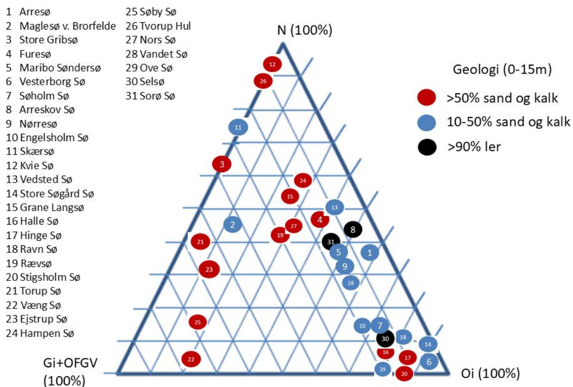
Figur 20: Ind-budgettet for 31 testsøer beregnet med DK-model2023.
