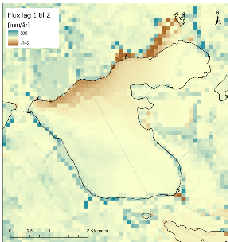
Figur 4: Grundvandsstrømning fra lag 1 til lag 2, positive værdier er nedadrettet flux (blå farver), i og omkring Furesø, Sjælland. Arealer med grundvandsindsivning til søen er vist med rød-brune farver.
