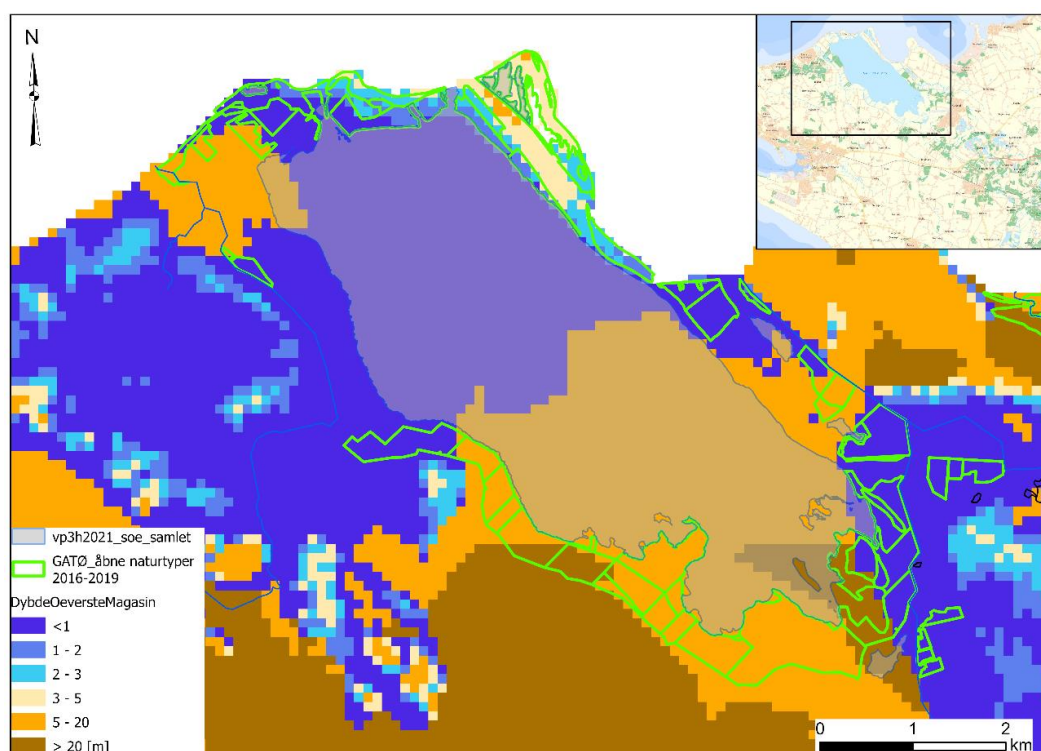
Figur 7: Dybde til øverste grundvandsforekomst for GATØ ved Kalundborg (grønne polygoner)
