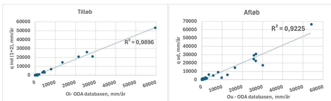
Figur 16: Modellerede versus målte vandføringer i tilløb (venstre) og afløb (højre) til målsatte søer.
