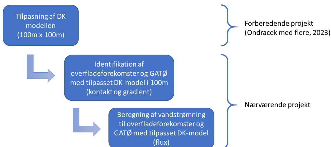
Figur 1: Projektsammenhænge mellem modellering af vandudvekslingen mellem grundvand-overfladevand og GATØ i VP3 regi (2022-2023) rapporteret i Ondracek med flere (2023), og nærværende projekts beregning af kontakt, gradient og flux med tilpasset DK-model for vandløb, søer og GATØ.
