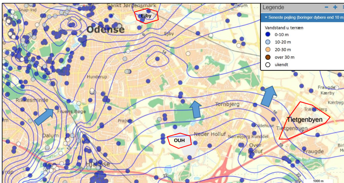
Figur 3.13. Oversigt over det forventede potentialebillede i de øvre grundvandsmagasiner i Odense SØ. Grundvandsstrømning sker vinkelret på konturkurverne mod laveste potentiale (m). Dvs. der sker en generel strømning fra syd mod nord. I vest ses en strømning fra bakkeområderne mod de lavereliggende områder i øst. Med punkter er vist målt vandstand i borerer dybere end 10 m (kilde: GEUS varmelagring web tool ). FVF fokusområder er vist med røde polygoner.
