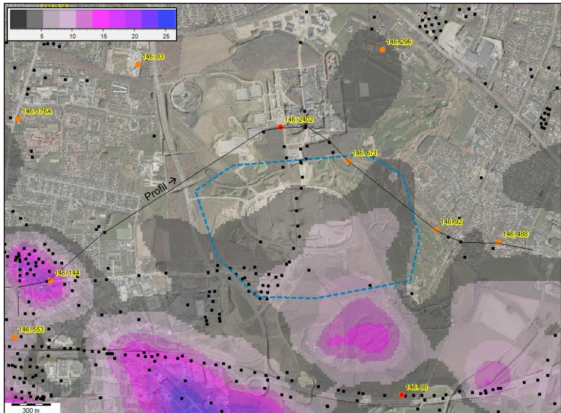
Figur 3.7. Oversigt over boringsdata og forventet udbredelse af regionalt kvartært sandmagasin (se legende øverst til venstre). Blå stiplede polygon angiver området ved det nye Odense Universitetshospital. Tværsnitsprofilen er vist på Figur 3.8.
