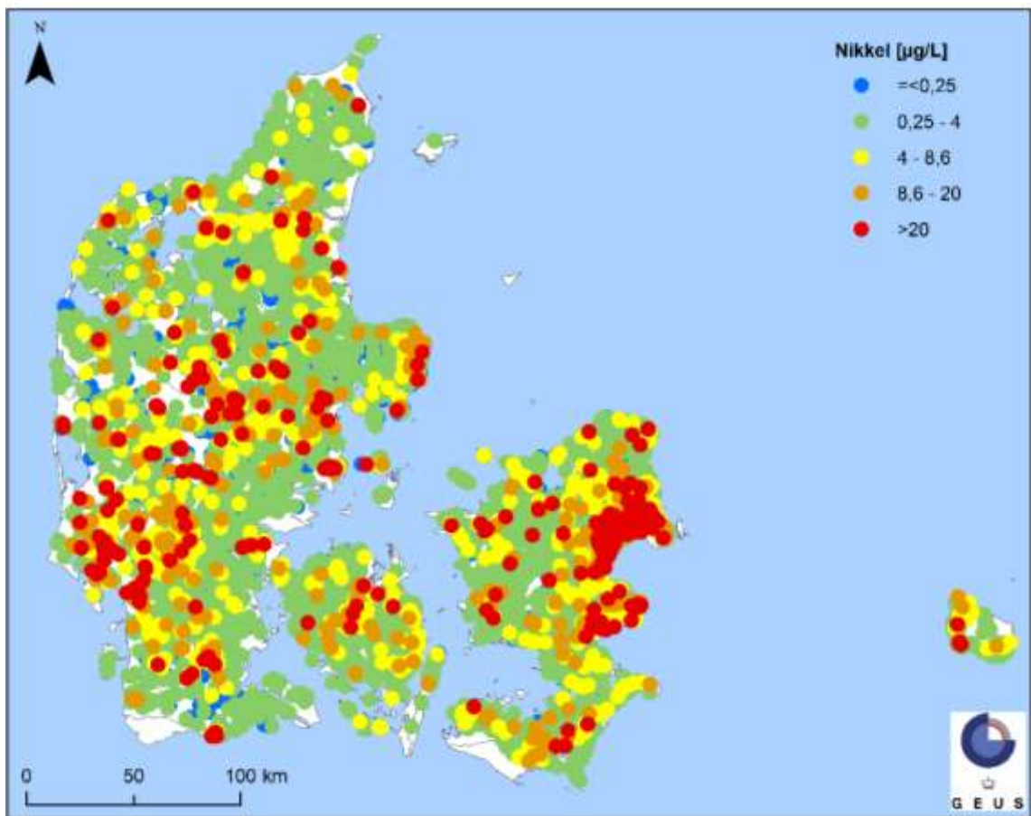
Figur E11 Nikkel i grundvand, middelværdier for perioden 2000-2013 (Data fra Thorling og Sørensen, 2014). Kravværdien for nikkel i drikkevand er 20 \mu\text{g/l} . Den højeste koncentrationsklasse er vist øverst.
