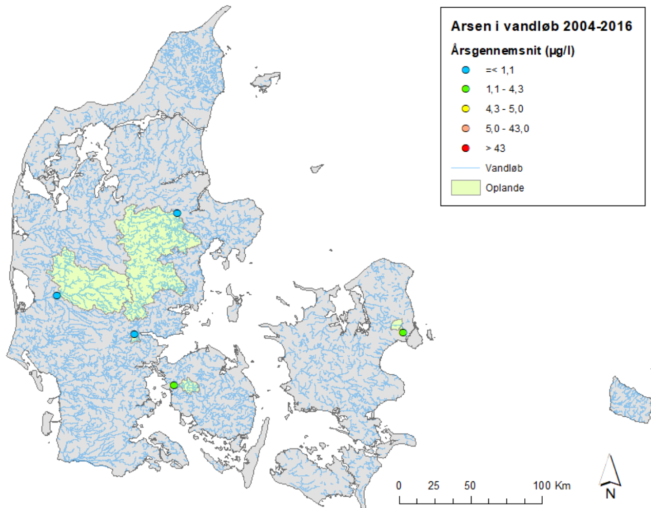
Figur F12: Arsen i vandløb i Danmark i perioden 2004-2016. Figuren viser årsgennemsnit for hver vandløbsstation udregnet på baggrund af metode 2 (NOVANA metoden) for hvert kalenderår. Der er i alt behandlet data fra 5 forskellige vandløbsstationer. I de tilfælde, hvor der er flere årsgennemsnit ved samme station er det årsgennemsnittet fra det seneste år der er vist.
