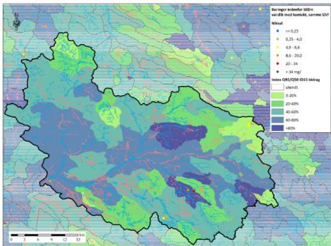
Figur K6: Placering af indtag i Skjern Å omlandet hvor der er målt efter nikkel, og hvor indtagene er placeret i en afstand på 500m eller mindre til en vandløbsstrækning med god kontakt, samt hvor indtagene er placeret i en grundvandsforekomst som har kontakt til et vandløb i ID15 omlandet, sammenstillet med Index Q95/Q50 pr ID15.
