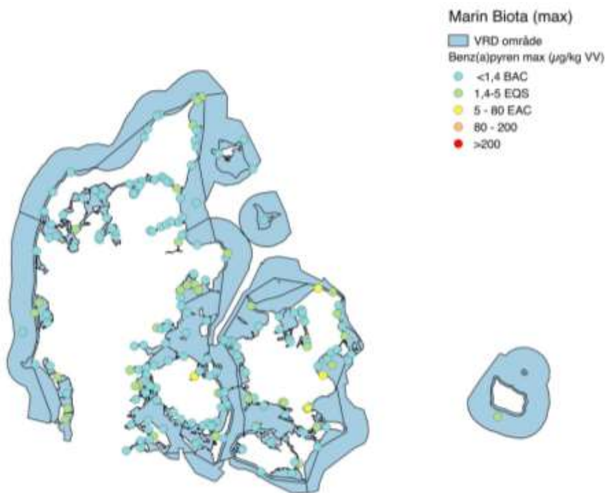
Figur G4: Benz(a)pyren i muslinger. Enkelte områder er over EQS (5 af 222 stationer ved Odense og omkring øst Sjælland), højest målte koncentration er 7,4 \mu\text{g/kg VV} .
