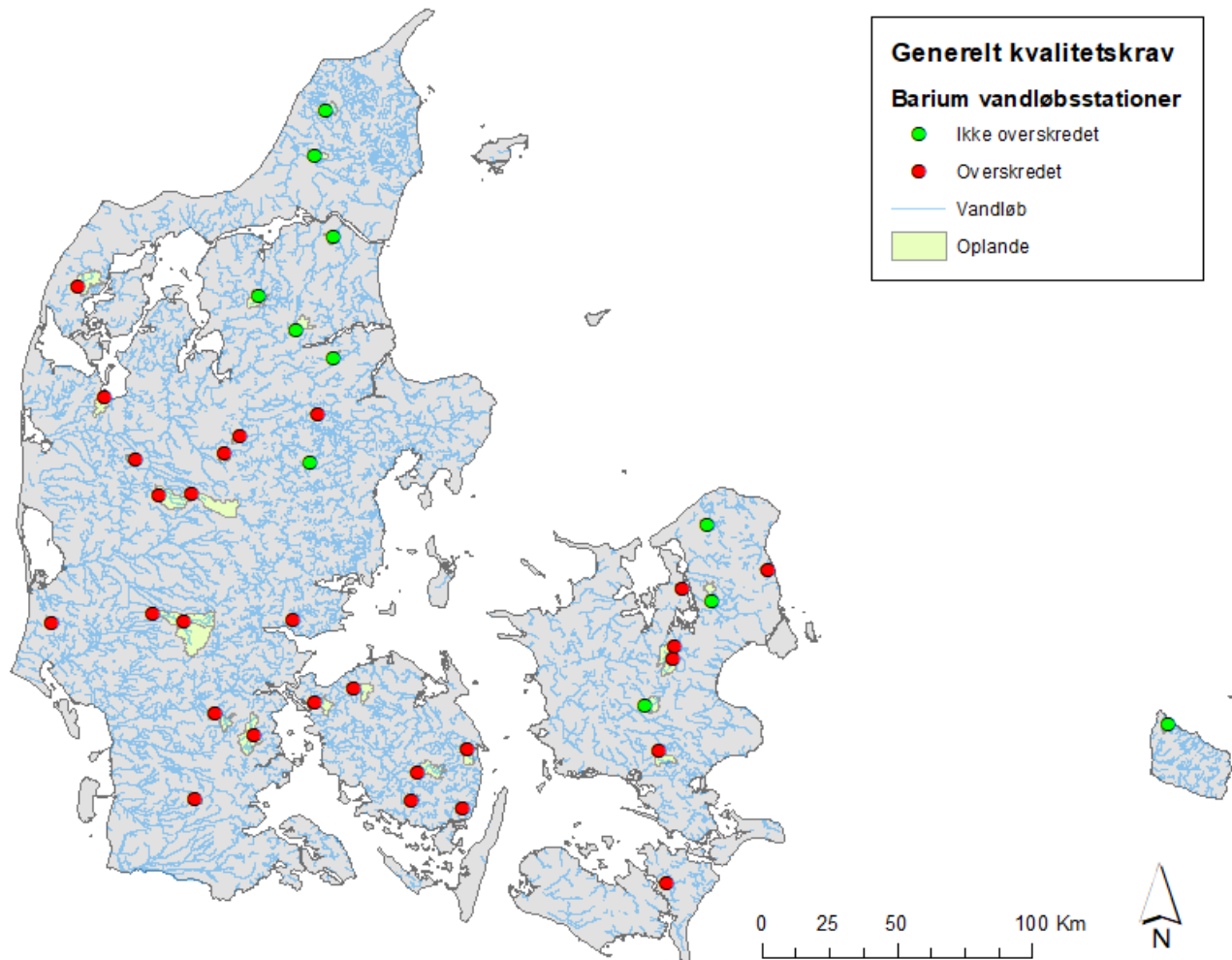
Figur F18: Den rumlige fordeling af årsgennemsnits-koncentrationer i forhold til det generelle kvalitetskrav på 34 µg/l for barium i vandløb.
