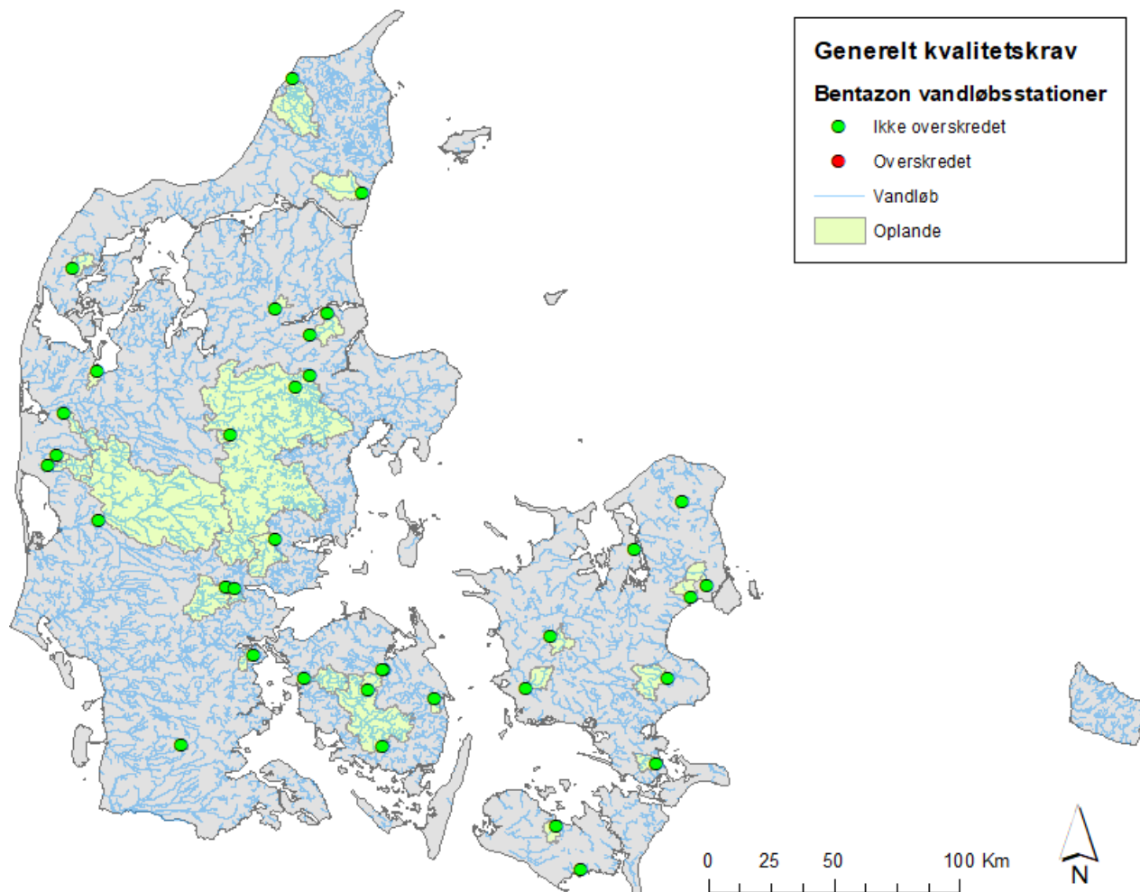
Figur F30: Den rumlige fordeling af årsgennemsnits-koncentrationer i forhold til det generelle kvalitetskrav på 45 µg/l for bentazon i vandløb.
