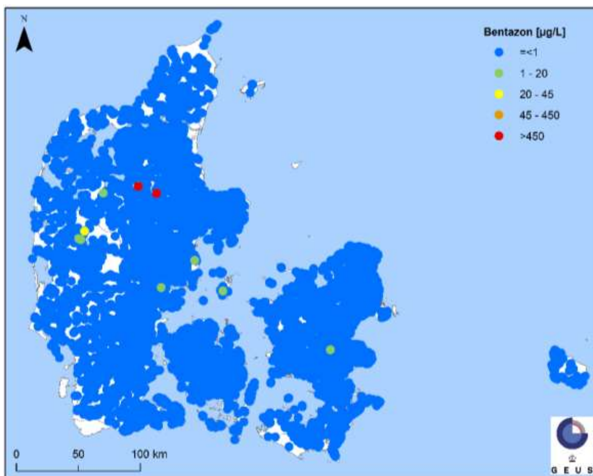
Figur E13 Bentazon ( \mu\text{g/l} ) grundvand middelværdier for alle datatyper. Gennemsnit for perioden 2007-2017.
