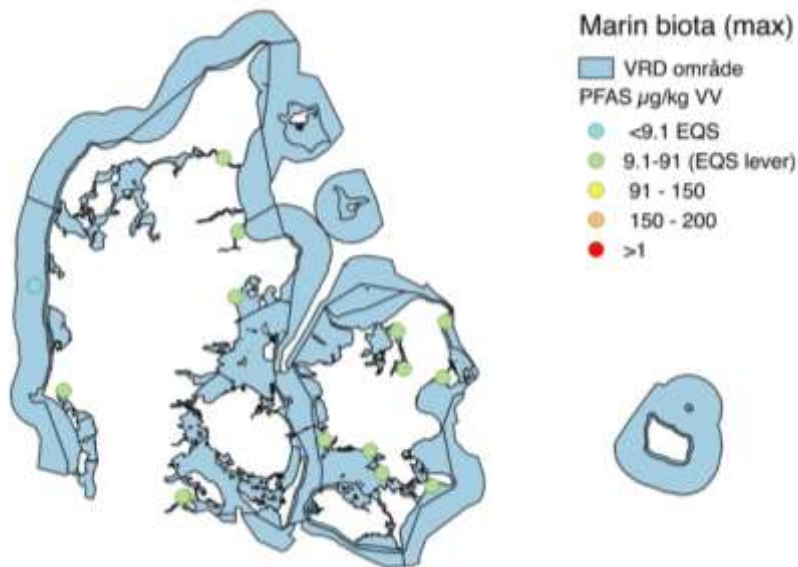
FigurG5: Summen af perfluorerede flammehæmmer(PFAS) i Fiske lever. PFOS udgør 26-71% af summen af PFOS'erne, den højeste værdi af PFAS er 41 mod 26 \mu\text{g/kg VV} PFOS.
