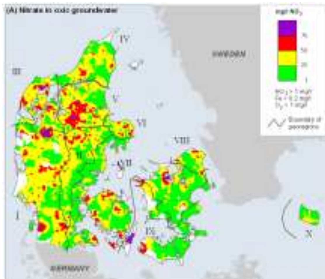
Figur E9. Georegioner og nitrat i iltet grundvand. Hansen med flere (2012).
