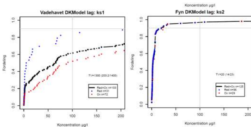
Figur C7: Fordeling for aluminium i hhv. iltet og reduceret "grundvand model" lag kvartært sand 1 og 2" i Vadehavsoplandet og på Fyn, (Thorling og Sørensen 2014). Kravværdien for aluminium i drikkevand er 100 µg/l.
