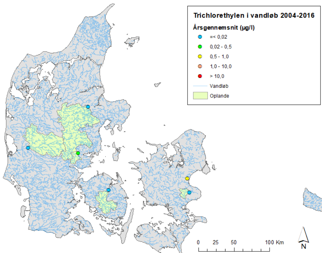
Figur F39: Trichloroethylen i vandløb i Danmark i perioden 2004-2016. Figuren viser årsgennemsnit for hver vandløbsstation udregnet på baggrund af metode 2 (NOVANA metoden) for hvert kalenderår. Der er i alt behandlet data fra 6 forskellige vandløbsstationer. I de tilfælde, hvor der er flere årsgennemsnit ved samme station er det årsgennemsnittet fra det seneste år der er vist.
