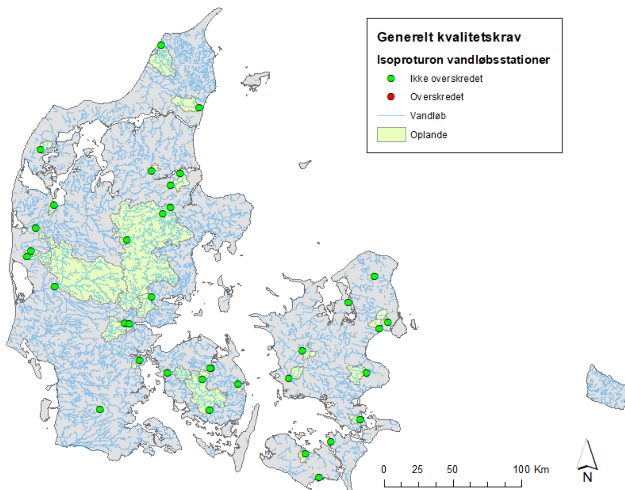
Figur F34: Den rumlige fordeling af målte årsgennemsnit-koncentrationer i forhold til det generelle kvalitetskrav på 0,3 µg/l for isoproturon i vandløb.
