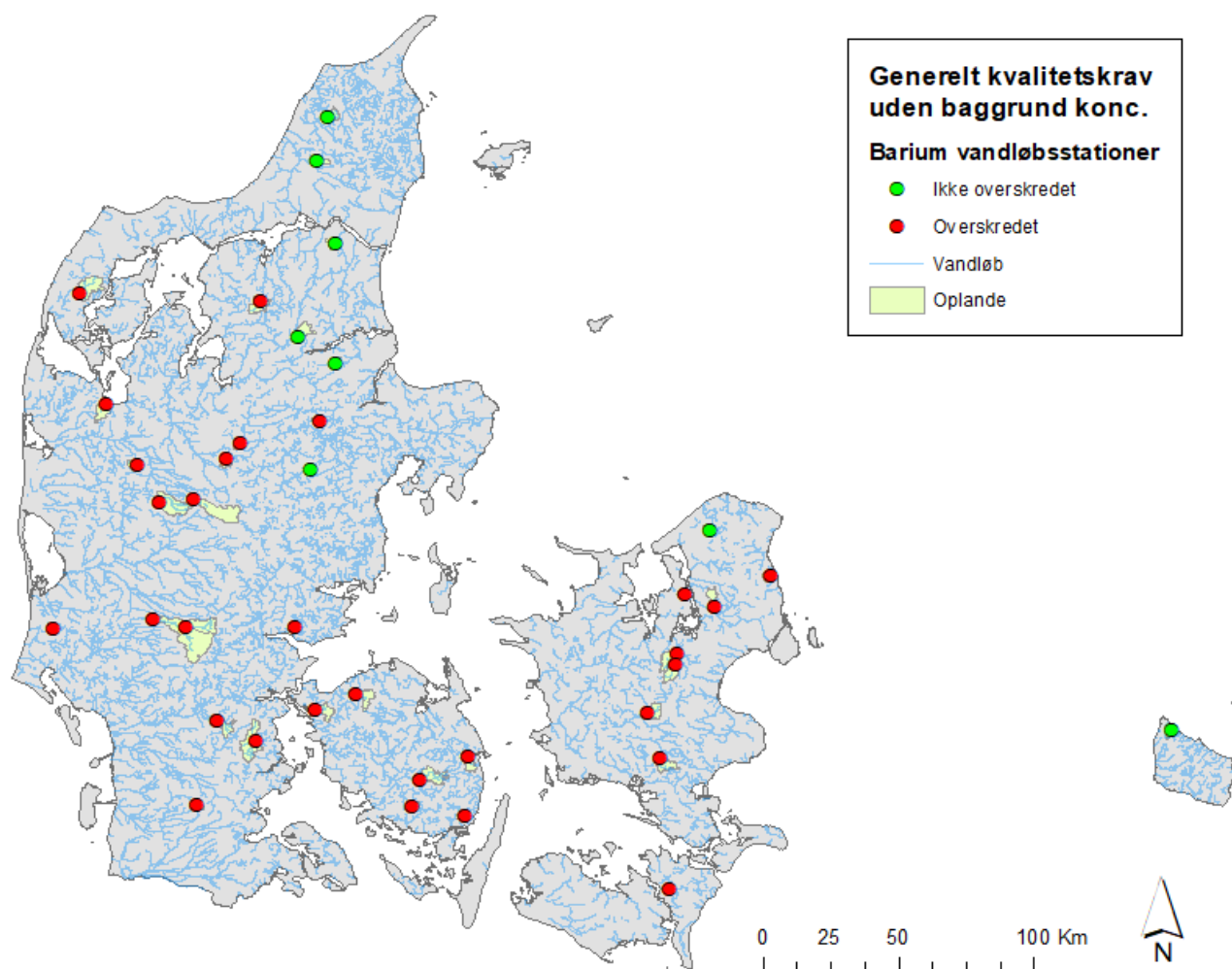
Figur F19: Den rumlige fordeling af årsgennemsnits-koncentrationer i forhold til det generelle kvalitetskrav uden hensyn til den naturlige baggrundskoncentration på 19 µg/l for barium i vandløb.
