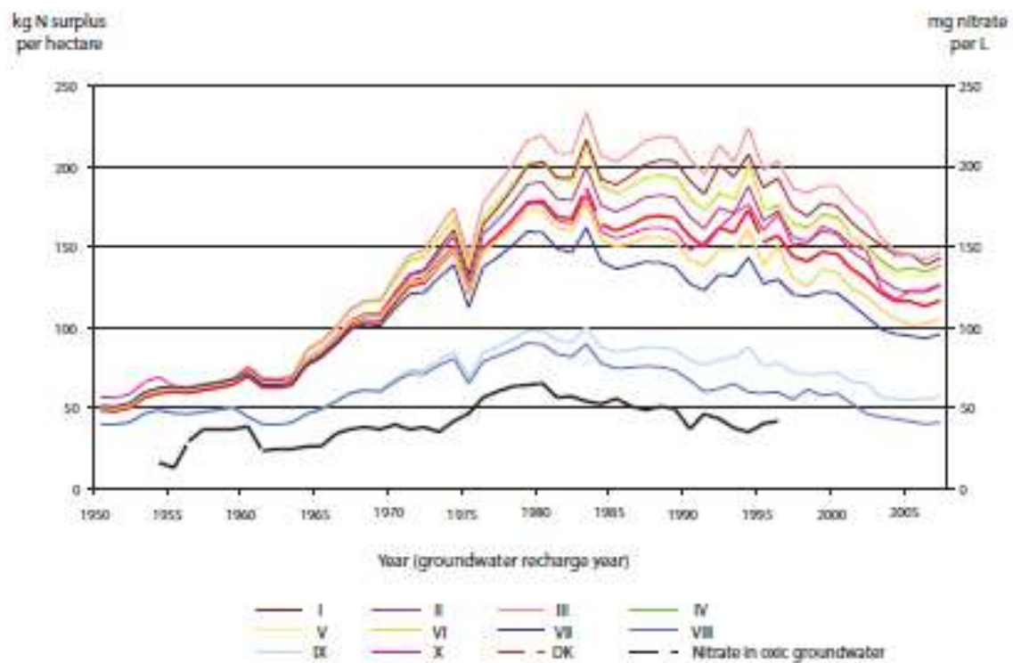
Figur E8. Kvælstofoverskuddet i georegioner i DK, og nitrat i iltet grundvand. (Hansen med flere, 2012)
