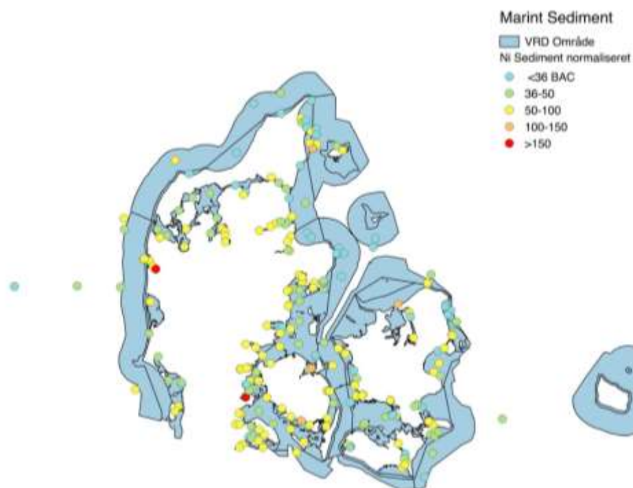
Figur B9: Nikkel i sediment, normaliseret til Li. Bemærk at der kun er en BAC defineret, så farveskalaen er tilpasset afrundede værdier.
