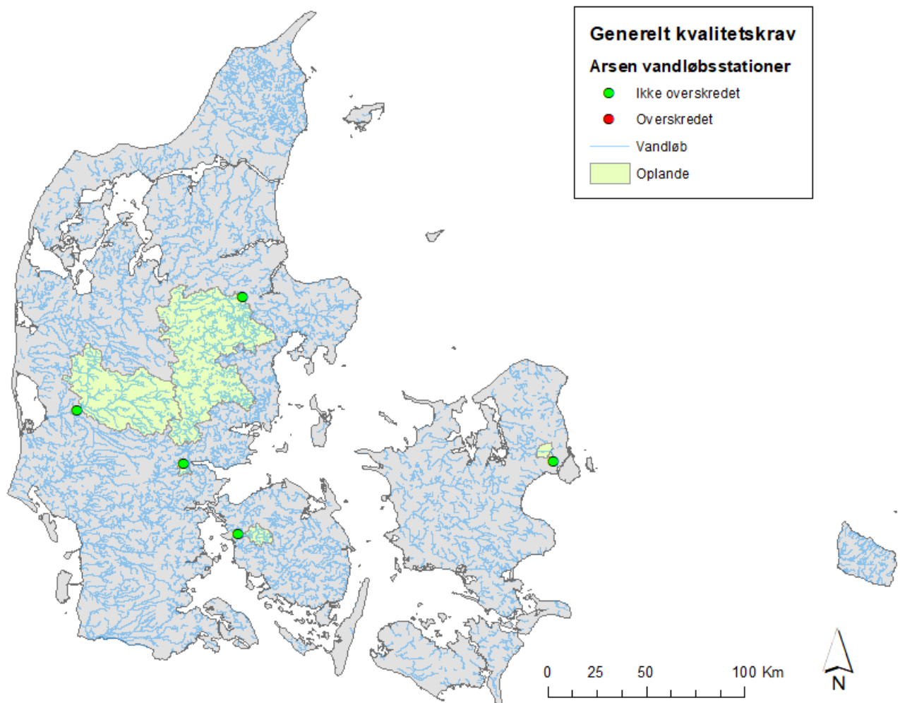
Figur F14: Den rumlige fordeling af årsgennemsnits-koncentrationer i forhold til det generelle kvalitetskrav på 4,3 µg/l for arsen i vandløb.
