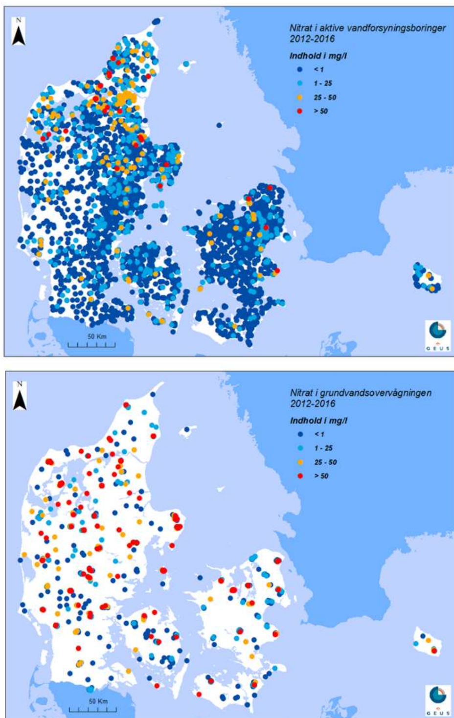
Figur E5 Nitratindholdet i grundvandet i 5.951 aktive vandværksboringer fordelt på fire koncentrations-klasser og 1236 GRUMO indtag. Kortet er baseret på gennemsnit per indtag for perioden 2012-2016. Den højeste koncentrationsklasse ligger øverst. (Thorling med flere, 2018).
