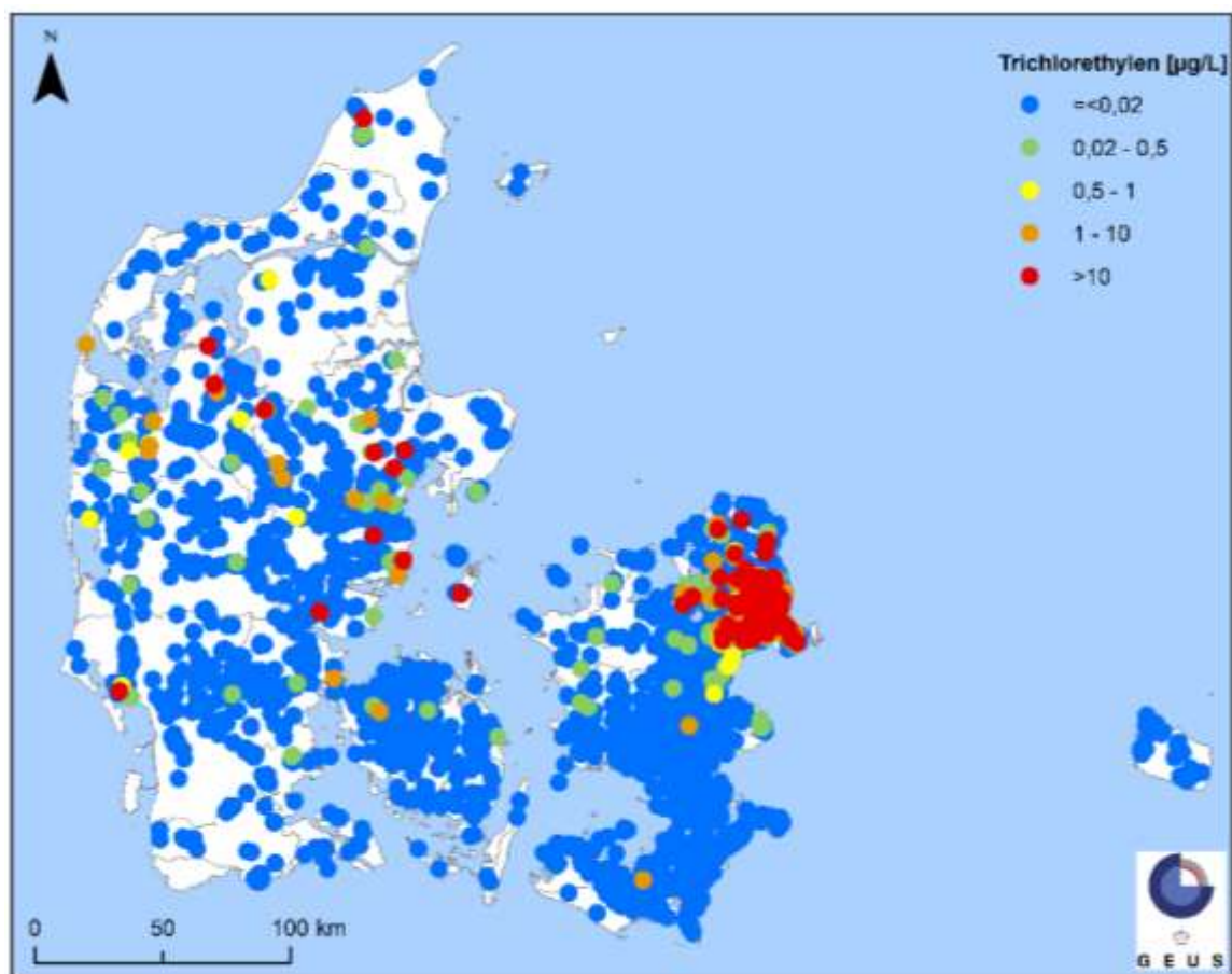
Figur E16 Trichlorethylen (µg/l) grundvand middelværdier for alle datatyper. Gennemsnit for perioden 2007-2016.
