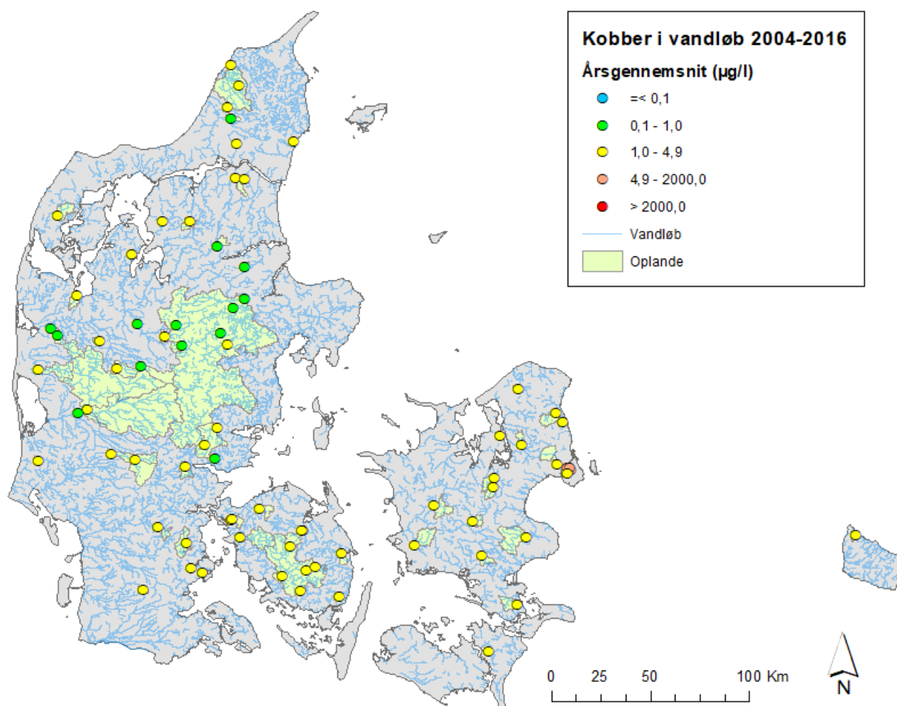
Figur F24: Kobber i vandløb i Danmark i perioden 2004-2016. Figuren viser årsgennemsnit for hver vandløbsstation udregnet på baggrund af metode 2 (NOVANA metoden) for hvert kalenderår. Der er i alt behandlet data fra 66 forskellige vandløbsstationer. I de tilfælde, hvor der er flere årsgennemsnit ved samme station er det årsgennemsnittet fra det seneste år der er vist.
