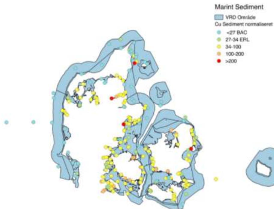
Figur B10: Kobber i sediment, normaliseret til Li.
