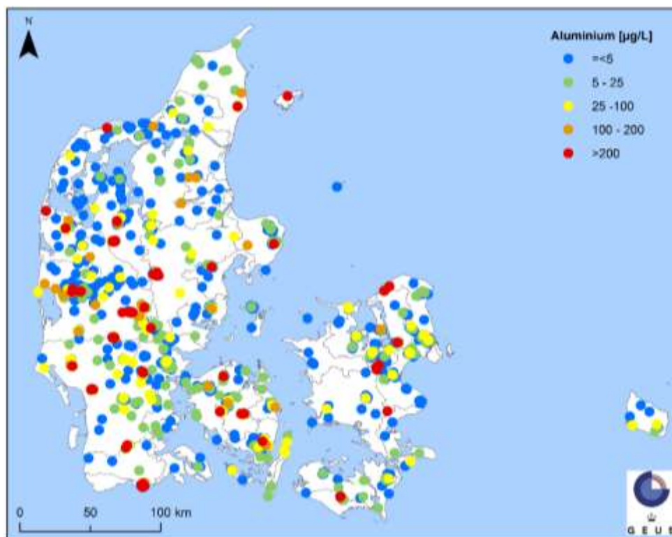
Figur C6: Aluminium i Grundvandsprøver. middelværdier for perioden 2000-2017. Den højeste koncentrationsklasse er vist øverst.
