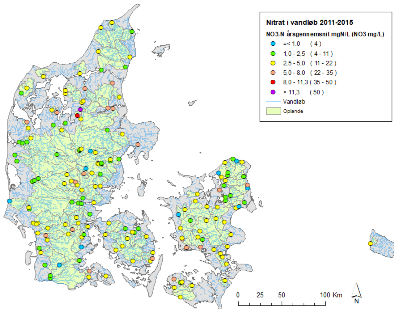
Figur F2: Nitrat i vandløb i Danmark i perioden 2011-2015. Figuren viser årsgennemsnit for de enkelte vandløbsstationer udregnet på baggrund af metode 2 (NOVANA metoden) for hvert kalenderår. Der er i alt behandlet data fra 171 forskellige vandløbsstationer. I de tilfælde, hvor der er flere årsgennemsnit ved samme station er det årsgennemsnittet fra det seneste år der er vist.
