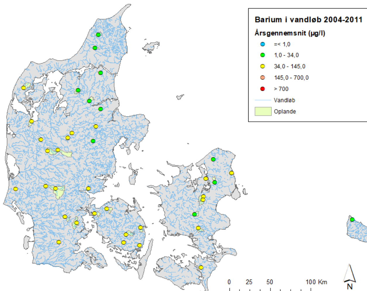
Figur F16: Barium i vandløb i Danmark i perioden 2004-2016. Figuren viser årsgennemsnit for hver vandløbsstation udregnet på baggrund af metode 2 (NOVANA metoden) for hvert kalenderår. Der er i alt behandlet data fra 38 forskellige vandløbsstationer. I de tilfælde, hvor der er flere årsgennemsnit ved samme station er det årsgennemsnittet fra det seneste år der er vist.
