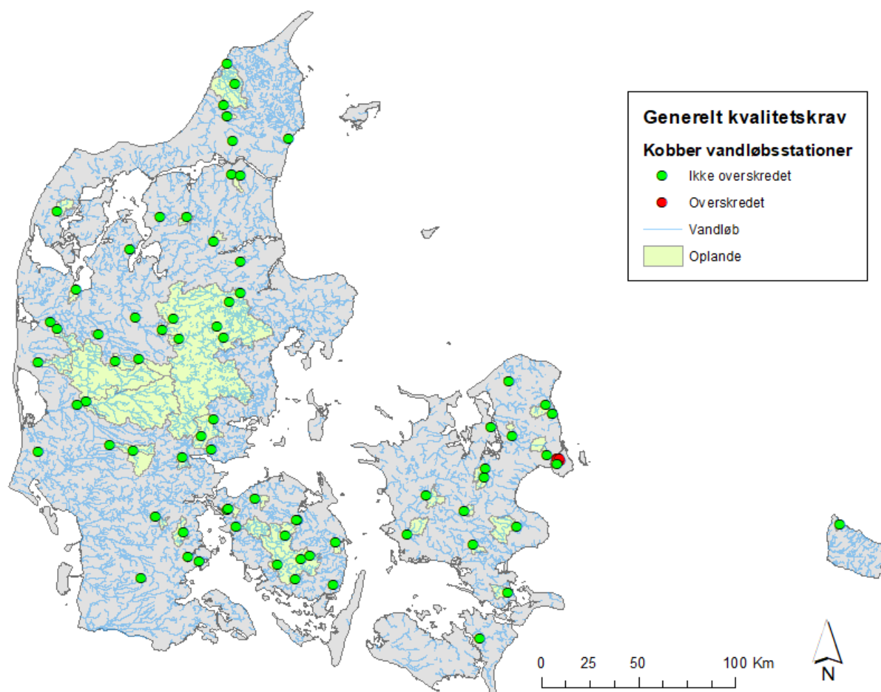
Figur F26: Den rumlige fordeling af årsgennemsnits-koncentrationer i forhold til det generelle kvalitetskrav på 4,9 µg/l for kobber i vandløb.
