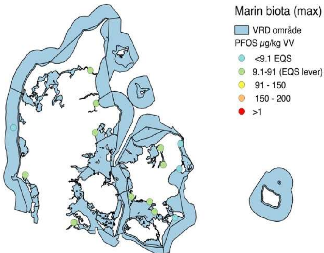
Figur 7.19: Perfluoroktansulfonsyre (PFOS) i fiskelever. EQS værdien er sat for hele fisk (9,1 \mu\text{g/kg VV} ), men der er dokumenteret en faktor ca. 17 mellem lever- og filetindhold af Perfluoroktansulfonsyre (PFOS), så en faktor 10 anvendes her som udgangspunkt for en "grøn" overgang.
