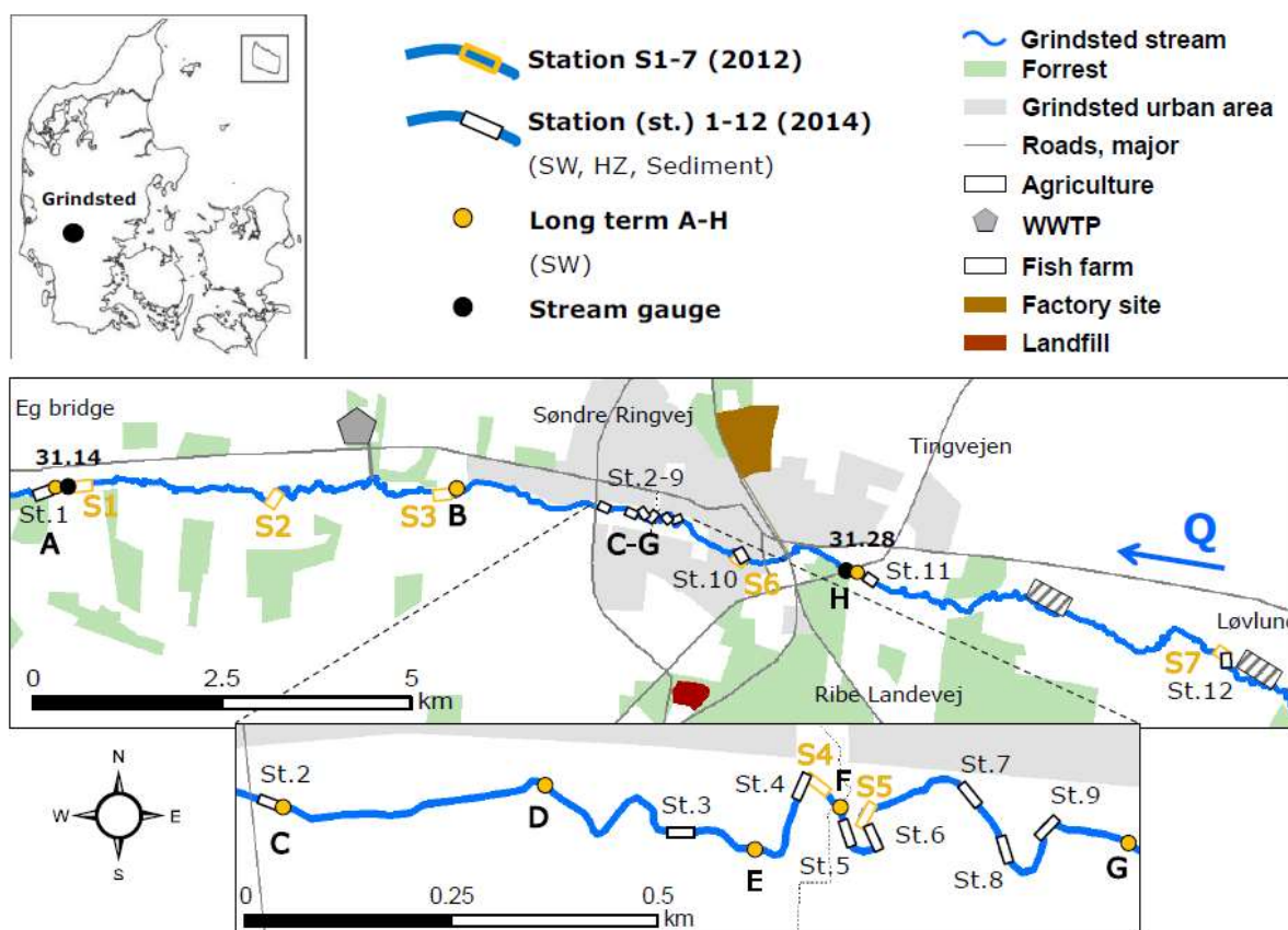
Figur 3.1: Måleopstillingen ved Grindsted Å, der er anvendt som et værkstedsområde for studier af forekomst og effekt af miljøfremmede stoffer (Sonne med flere, 2017b).
