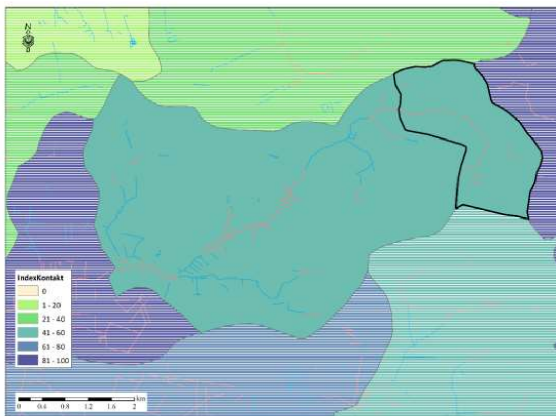
Figur 9.18: Index over kontakten mellem FOT vandløb og grundvandsforekomster. FOT vandløb vist med to farver: rød for strækninger med potentiel kontakt til grundvandsforekomst og blå for strækninger med potentiel ringe kontakt til grundvandsforekomsten. Bemærk at de potentielle kontakt for vandløbene udelukkende er vurderet ud fra 3m kravet.
