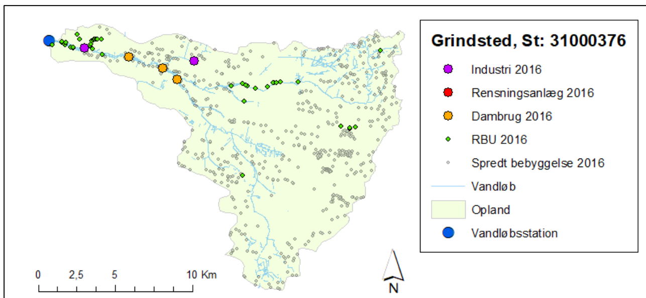
Figur 9.11: Placeringen af de forskellige overfladepunktkilder i Grindsted Å-opland år 2016. RBU: regnvandsbetinget udløb.
