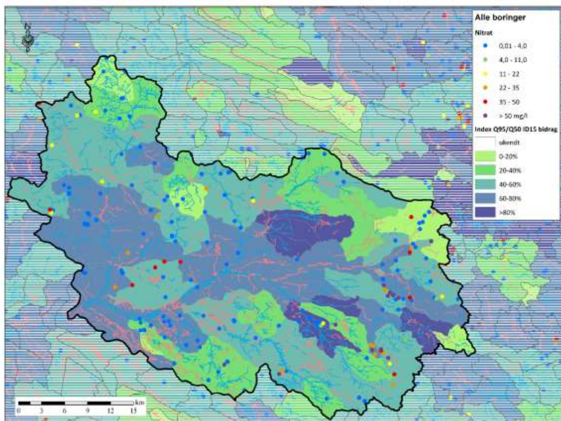
Figur 9.8: Placering af alle indtag hvor der er målt nitrat (mg/L) sammenstillet med index Q95/Q50 pr. ID15-opland. Bemærk at kontakten mellem GVF og vandløbsbund er baseret på PK.
