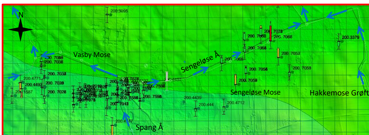
Figur 9 Kalibreret model og fejl på trykniveau (head) observationer. Størrelsen af søjlerne repræsenterer fejlen mellem simuleret og observeret trykniveau i de givne boringer. Differensen imellem simuleret og observeret trykniveau er inddelt i tre farve kategorier: differens på 0-75 cm (grøn), differens på 75-150 cm (gul) og differens > 150 cm (rød). Potentialelinjer er optegnet på baggrund af Store Pejledag 2016 målingerne. Nederst er vist et zoom af området ved selve moserne.
