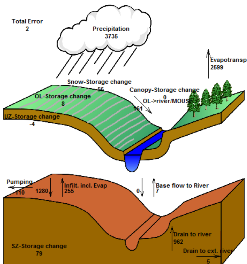
Figur 8 Illustrationen viser de led i vandbalancen der indgår i DK-modellens opsætning. Vandbalance for Riggilde modellens område indeholder de samme vandbalanceled som vist i figuren og er udtrukket fra DK-modellen for perioden 2011-2015. Alle tal-værdier er opgjort i mm og er akkumuleret over perioden 2011-2015. Figuren er modificeret fra /11/.
