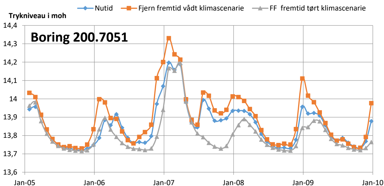
Figur 17 Simulererede vandstande i kalkmagasinet under moserne og i moseaflejringerne beregnet med Rigmilde modellen i et nutidigt klima og i et fremtidigt vådt og et fremtidigt tørt klima. 200.126 repræsenterer trykniveauet (vandstanden) i det primære kalk magasin, mens 200.7051 (SM1-3.5 i Sengeløse Mose med filter i 3,5 meters dybde) repræsenterer trykniveauet i moseaflejringerne.
