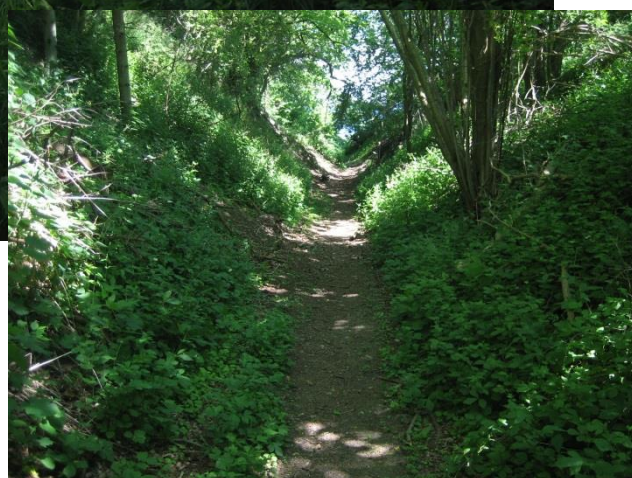
Figur 78. Kulstirenden er den eneste slugt, som naturligt fører ned til stranden ved Stevns Klint. Slugten har en nordøstlig retning, som kan sammenstilles med retningen af ekstensionelle sprækker.
