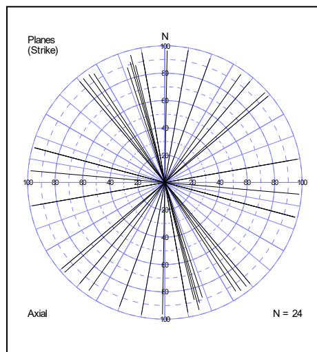
Figur 62. Sprækkeretningerne i Harvig præsenteret i et rosedigram diagram. Bemærk den dominerende shearretning 140^\circ – 170^\circ . Desuden ses det konjugerede sæt 10^\circ – 105^\circ .
