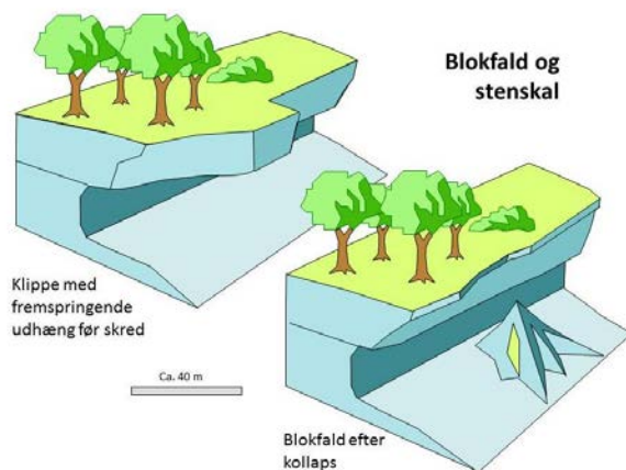
Figur 20. To blokdiagrammer, som illustrerer situationen før og efter kollapse af klintblokken ved Klintegård. Skreddet må primært betragtes som et blokfald, men med den konkavt hældende brudflade må skreddet samtidig også være foregået som stenskal, hvor enkelte flager har løsrevet sig.
