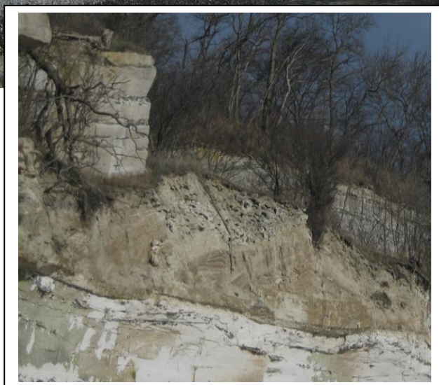
Figur 34. Overjordsdynger med fyldmateriale i det gamle kalkbrud ved Højeruplund giver anledning til bekymring, da løse sten og blokke konstant falder ned fra disse. På fotoet herover ses, hvordan fyldet ligger i dynger i bunden af det langstrakte kalkbrud. Til højre et nærbillede af en jorddyng med tydelig skrålejrning fra opfyldet. Der må advares mod stenras fra disse dynger.
