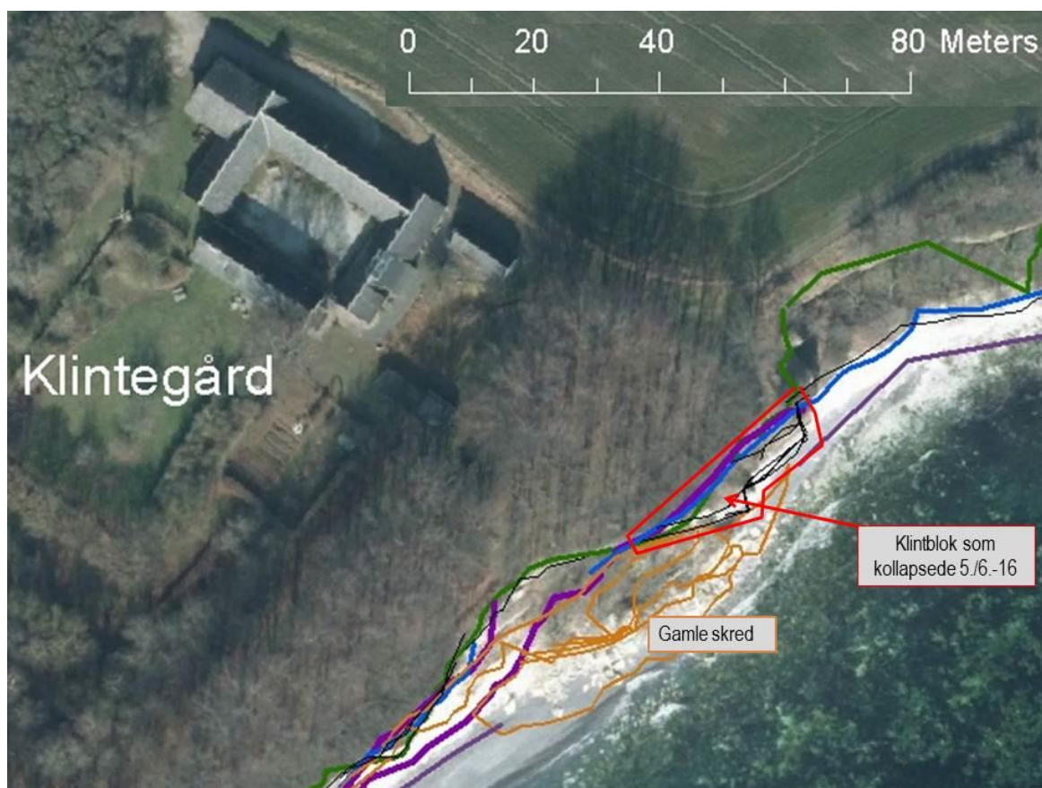
Figur 15. Et mere detaljeret udsnit af lodbilledet, som viser den kortlagte kalkbloks omrids. Bemærk at den blå streg angiver beliggenhed af kridtvæggen under overhænget. De sorte streget angiver bryozokalk væggen. Den grønne streg er toppen af klinten, mens de brune streger angiver skredkeglen dannet ved det gamle skred, som ifølge mundtlig overlevering skulle være sket for ca. 25 år siden.
