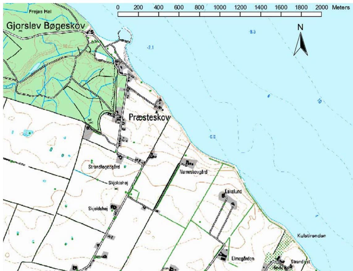
Figur 80. Kort over den nordligste del af Stevns Klint fra Kulstirønden til Bøgeskov havn. Området er her betegnet Præsteskov, som består af en nordlig del bestående af en morænelers klint, og en sydlig del som består af en klint domineret af skrivekridt. Skellet mellem de to typer klint er omtrentlig beliggende ud for Nørreskovgård.
