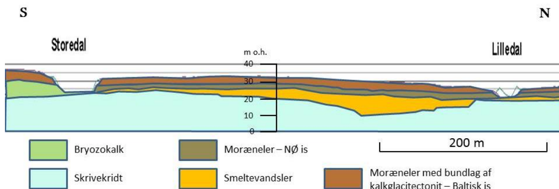
Figur 50. Geologisk tværprofil af området mellem Storedal og Lilledal, hvor den tykkeste mængde af kvartære aflejringer optræder på Stevns Klint. Stedet med den tykkeste mængde af smeltevandsler (blåler) er det sted, hvor den største erosion langs Stevns Klint forekommer. Skreddene her er dog ikke fjeldskred men derimod jordskred. Bemærk at profilet har en overhøjning på 1:2.
