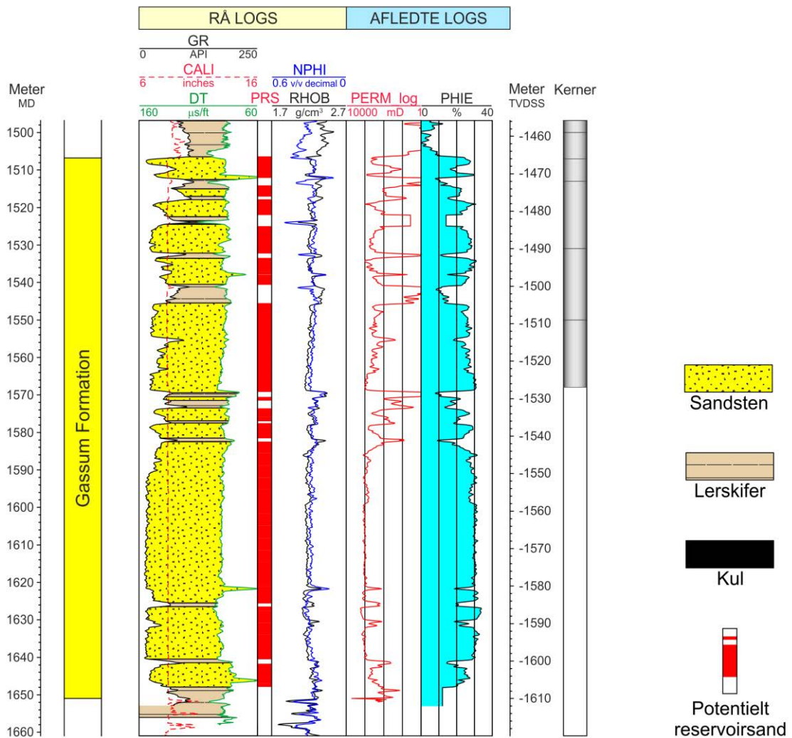
Figur 9: Petrofysisk log-tolkning af Gassum Formationen i Stenlille-1 inklusiv en tolkning af lithologien. Lithologi-kolonnen er afgrænset af gamma (GR) og sonic (DT) loggene. Sektioner med Potentielt reservoirsand (PRS) er markeret med rødt fyld. Porøsitetsestimatet (PHIE) er fremhævet med lyseblåt fyld, og permeabilitets-estimatet (PERM_log) er plottet som en rød kurve. Logforkortelserne er forklaret i Tabel 5.4. Formationen er i boringen vist med dens vertikale tykkelse. MD: Målt dybde fra referencepunkt på boreplatform, TVDSS: Vertikale dybde under havniveau.
