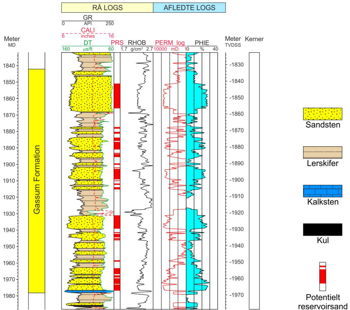
Figur 7: Petrofysisk log-tolkning af Gassum Formationen i Margretheholm-1/1A inklusiv en tolkning af lithologien. Lithologi-kolonnen er afgrænset af gamma (GR) og sonic (DT) log-gene. Sektioner med Potentielt reservoirsand (PRS) er markeret med rødt fyld. Porøsitets-estimatet (PHIE) er fremhævet med lyseblåt fyld, og permeabilitets-estimatet (PERM_log) er plottet som en rød kurve. Logforkortelserne er forklaret i Tabel 5.4. Formationen er i boringen vist med dens vertikale tykkelse. MD: Målt dybde fra referencepunkt på boreplatform, TVDSS: Vertikale dybde under havniveau.
