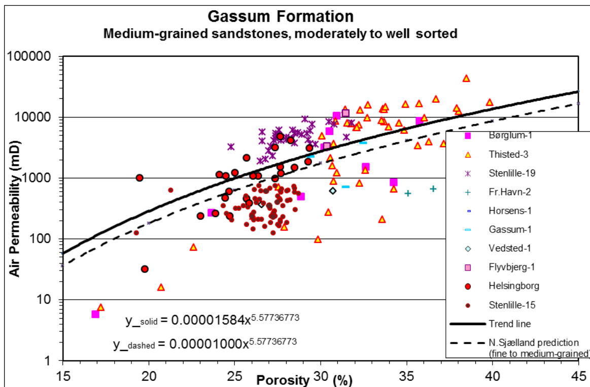
Figur 11: Generaliseret sammenhæng mellem porøsitet og permeabilitet estimeret ud fra kerneanalyse data, dvs. målinger af porøsitet og permeabilitet på små plug prøver, primært fra mellemkornede sandstenslag i Gassum Formationen. Den fuldt optrukne linje repræsenterer tendenslinjen for de plottede datapunkter. Den stiplede linje antages at være gældende for Nordsjælland og tilgrænsende områder, herunder også Roskilde-området. Forskellen på forløbet af de to tendenslinjer beror på, at Gassum reservoiret på Sjælland ikke udelukkende består af mellemkornet sandsten, men er en blanding af både fin- og mellemkornet sandsten. Usikkerheden på porøsitet-permeabilitets relationen er beskrevet og perspektiveret i teksten.
