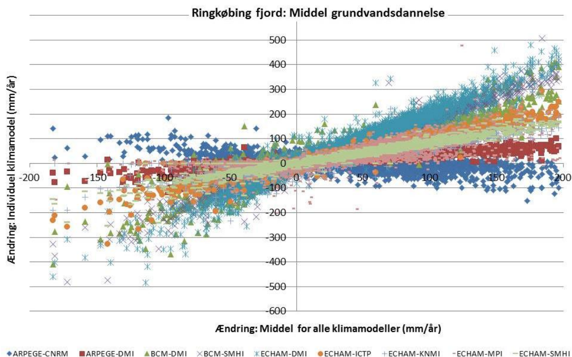
Fig. A2.3 Resultater for Ringkøbing fjord inputusikkerheder: ændring i middel grundvandsdannelse, i mm/år, 2021-2050 i forhold til 1961-1990.
