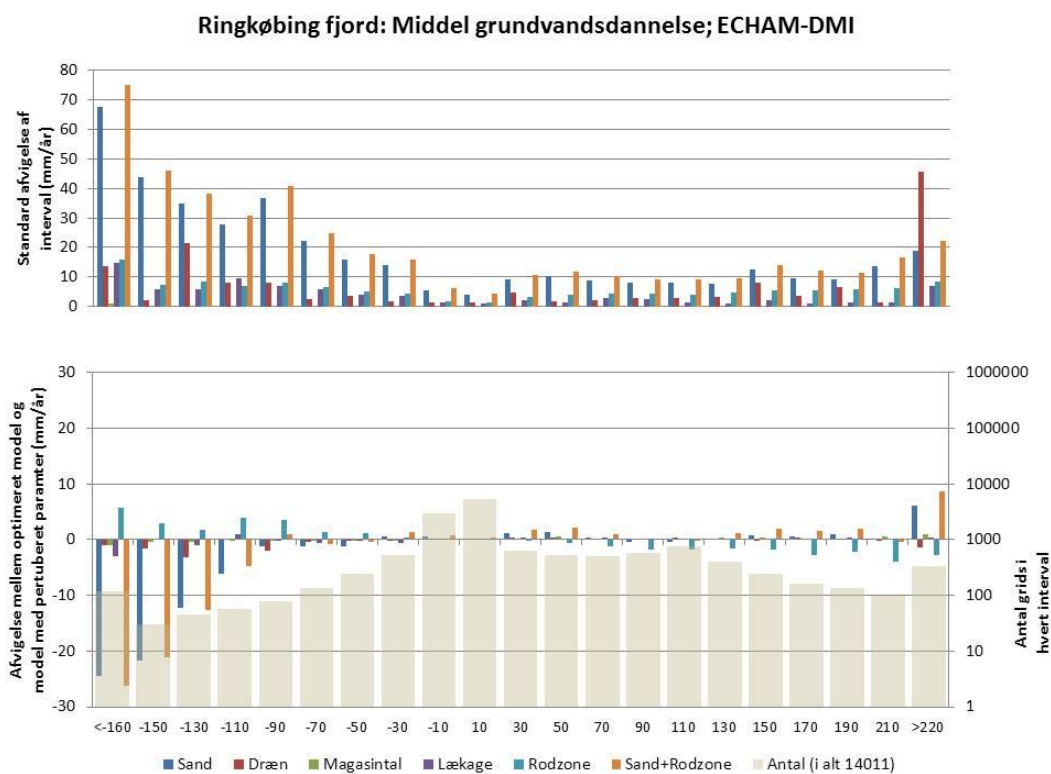
Fig. A2.11 Resultater for Ringkøbing fjord parameterusikkerheder: Ændring i middel grundvandsdannelse i mm/år, 2021-2050 i forhold til 1961-1990.
