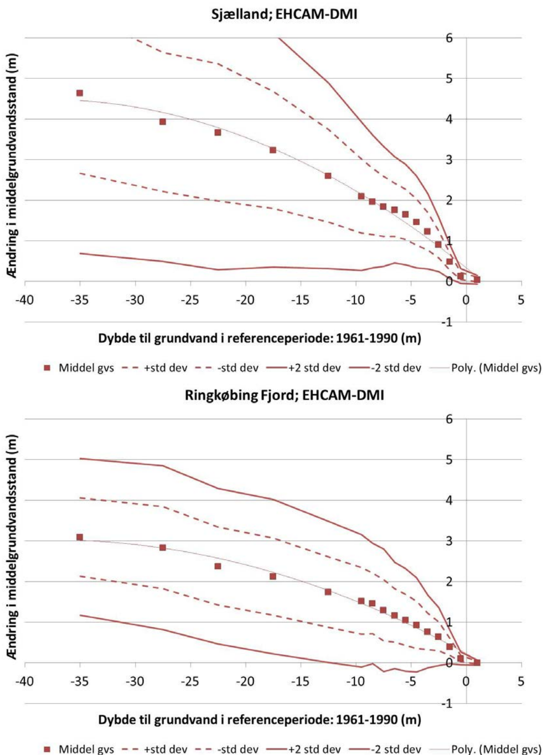
Figur 4.6 Resultater for Sjælland og Ringkøbing Fjord oplandet. Ændring i middel grundvandsstand for Våd klimamodel (EHCAM/DMI) som funktion af dybden til det øvre (regionale) grundvandsspejl. Øverst Sjælland, Nederst Ringkøbing Fjord opland
