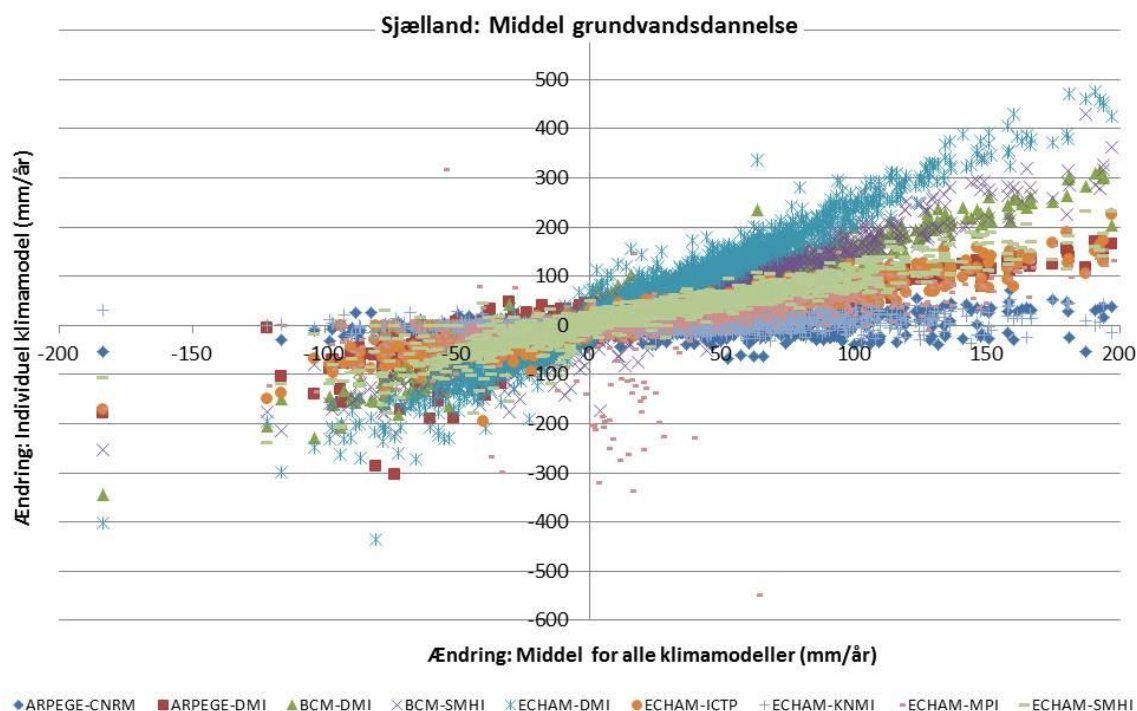
Fig. A2.7 Resultater for Sjælland inputusikkerheder: ændring i middel grundvandsdannelse, i mm/år, 2021-2050 i forhold til 1961-1990.
