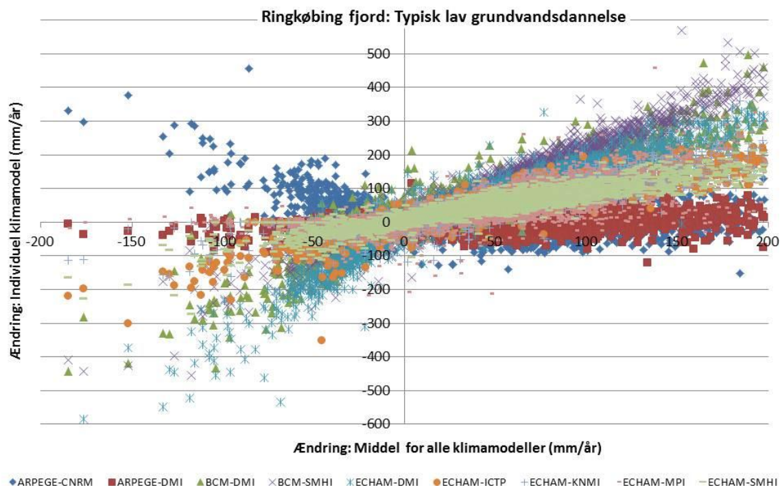
Fig. A2.4 Resultater for Ringkøbing fjord inputusikkerheder: ændring i typisk lav grundvandsdannelse, i mm/år, 2021-2050 i forhold til 1961-1990.
