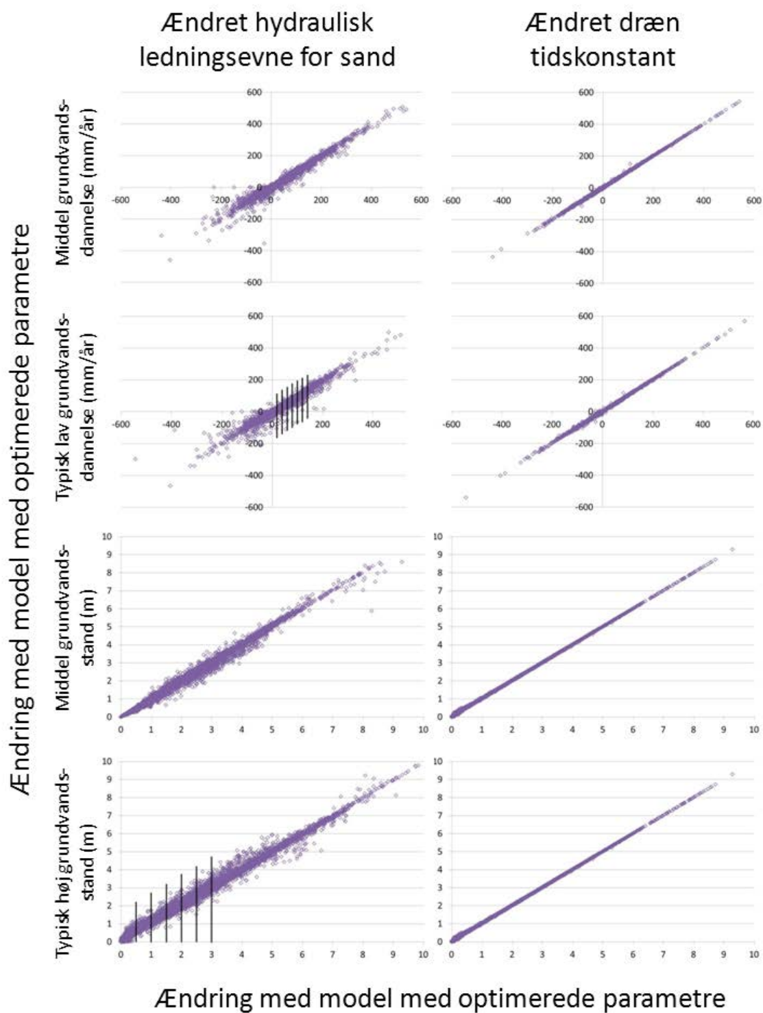
Figur 4.4 Resultater for Sjælland. I figuren til venstre er vist parameterusikkerheder, hvor x-aksen viser ændringer jf. optimeret DK-model for Sjælland og y-aksen viser ændringer jf. perturberet hydraulisk ledningsevne for sand (svarende til nedre konfidensgrænse). Ovenfra og ned er i venstre kolonne vist ændring i middel grundvandsdannelse, typisk lav grundvandsdannelse, middel grundvandsstand og typisk høj grundvandsstand ud fra domænets samtlige grid. Tilsvarende er i højre kolonne vist de samme udtræk men for parameteren 'dræntidskonstant'.
