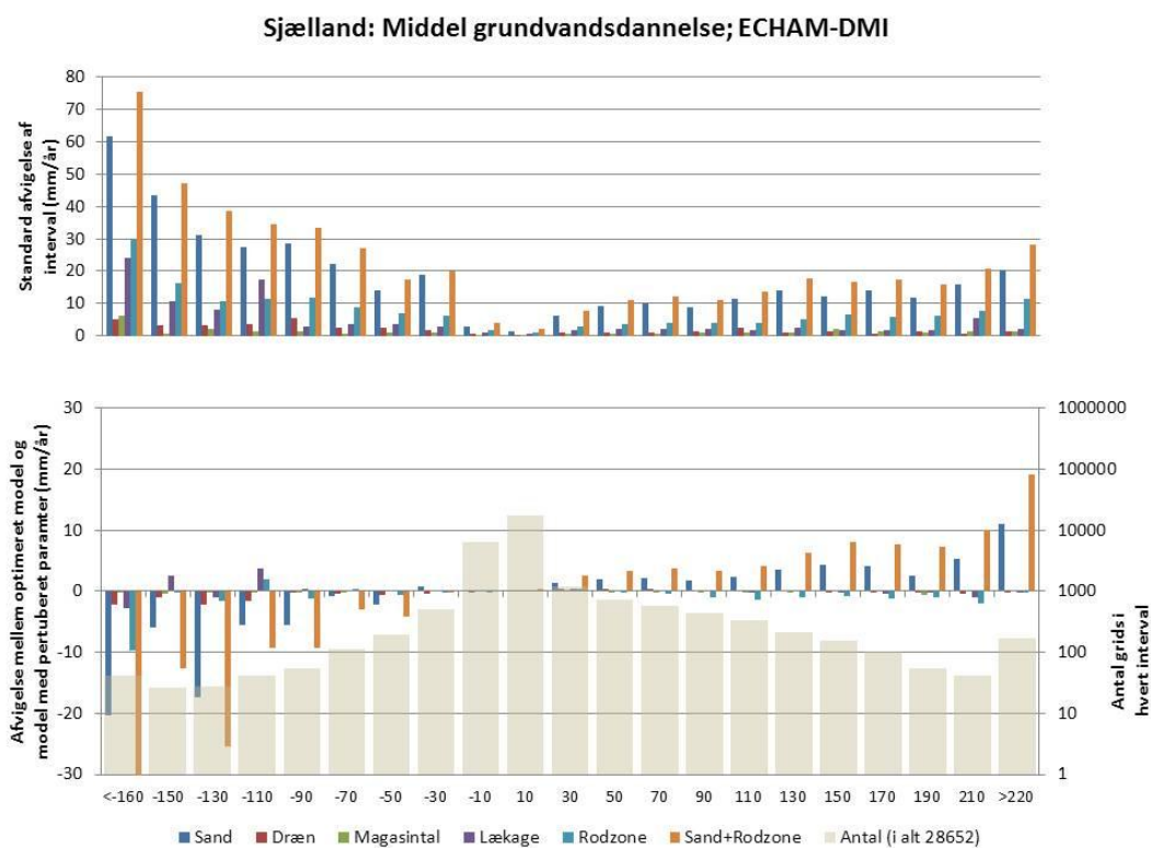
Fig. A2.15 Resultater for Sjælland parameterusikkerheder: Ændring i middel grundvandsdannelse i mm/år, 2021-2050 i forhold til 1961-1990.
