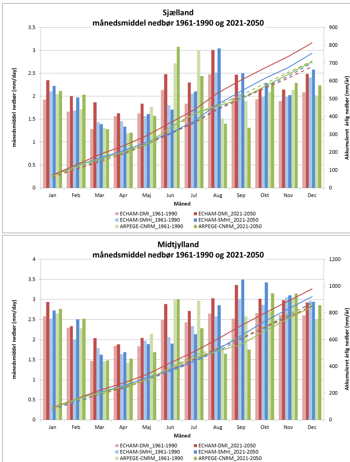
Figur 4.7 Ændringer i månedsnedbør for de tre udvalgte klimamodeller (ECHAM-DMI, ECHAM-SMHI og ARPEGE_CNRM) for referenceperioden 1961-1990 (tonede søjler) og fremtidsperioden 2021-2050 (udfyldte søjler). Desuden er vist akkumulerede værdier på stiplede kurver (1961-1990) og optrukne linjer (2021-2050).
