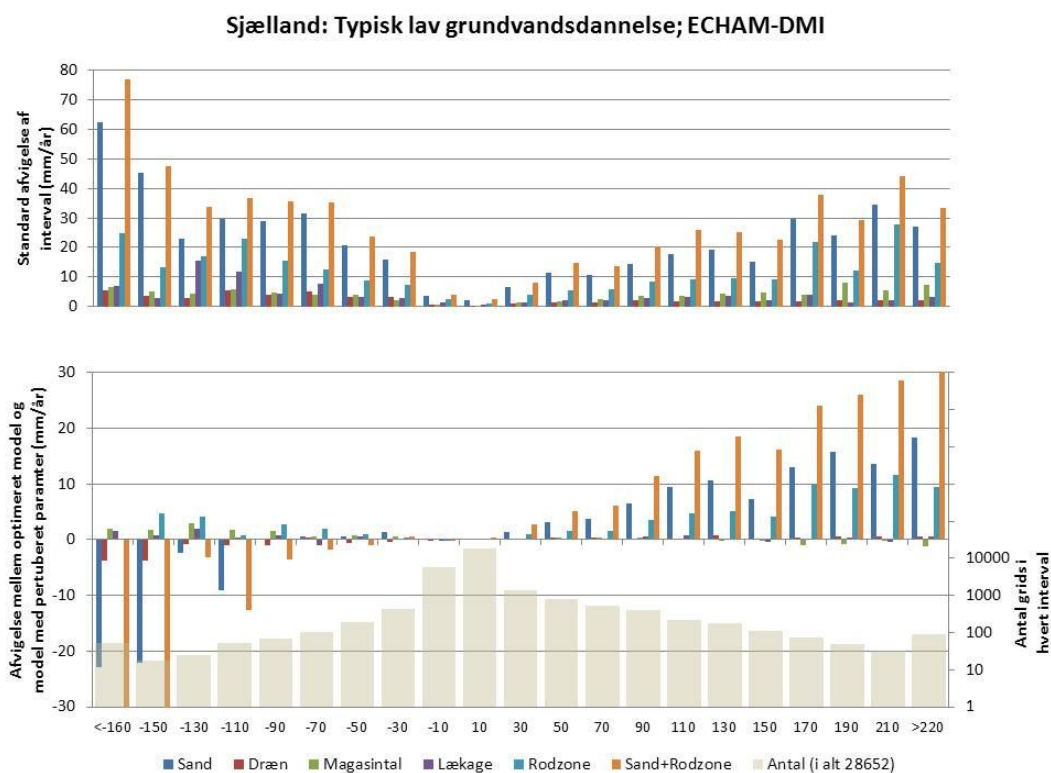
Fig. A2.12 Resultater for Sjælland parameterusikkerheder: Ændring i typisk lav grundvandsdannelse i mm/år, 2021-2050 i forhold til 1961-1990.
