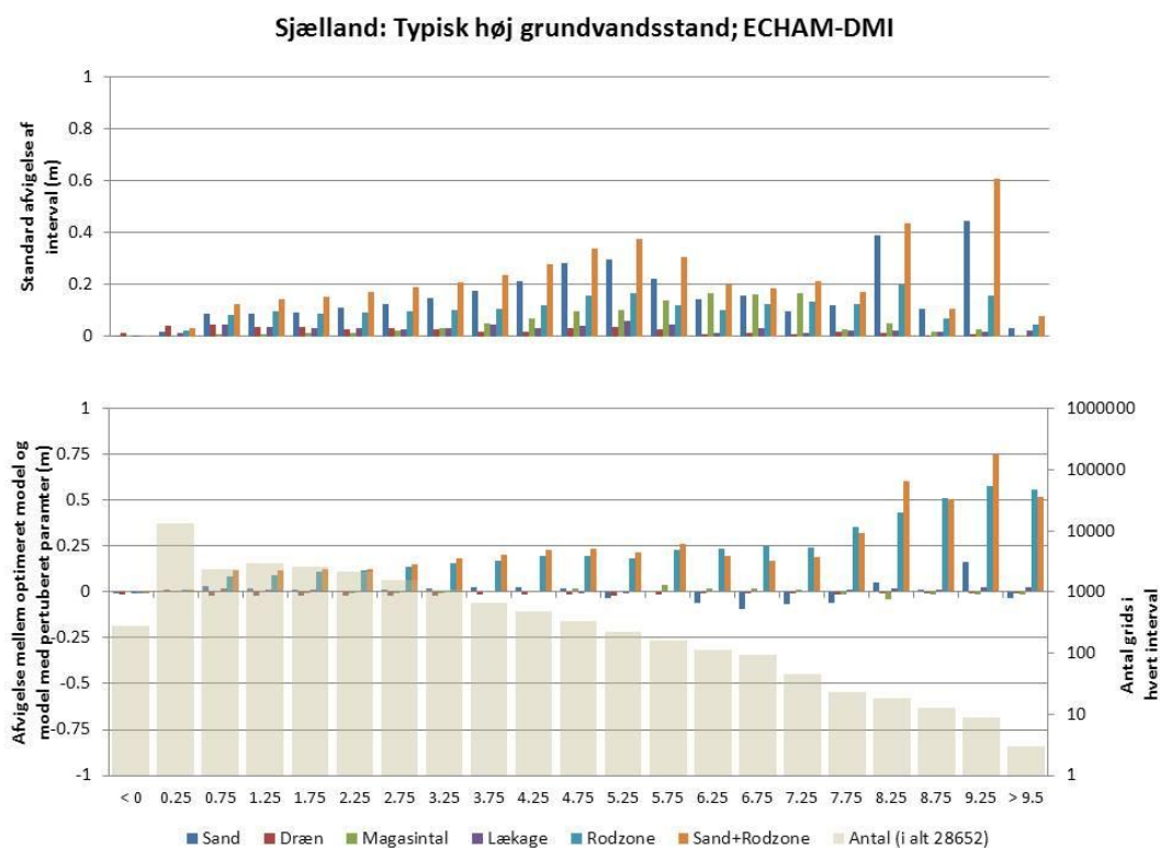
Fig. A2.14 Resultater for Sjælland parameterusikkerheder: Ændring i typisk højgrundvandsstand i m, 2021-2050 i forhold til 1961-1990.
