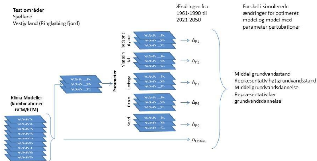
Figur 3.8 Usikkerhedsvurdering. Først gennemregnes simulerede ændringer for de fire leverancer i to testområder med de ni GCM/CRM kombinationer (KM1 – KM9 for Sjælland og Ringkøbing Fjord oplandet). Herefter udvælges de tre kombinationer der giver våd, median og tør fremskrivning og udsækker inputusikkerheden (KM_A - våd, KM_B - median og KM_C – tør). For de udvalgte parametre er der ud fra bestemte konfidensgrænser for Sjælland med PEST gennemført en perturbation jf. nedre konfidensgrænse (med bestemmelse af \Delta_{p1} , \Delta_{p2} ... \Delta_{p5} ) med henblik på sammenligning med betydning af inputusikkerhed ( \Delta_{Optim} )
