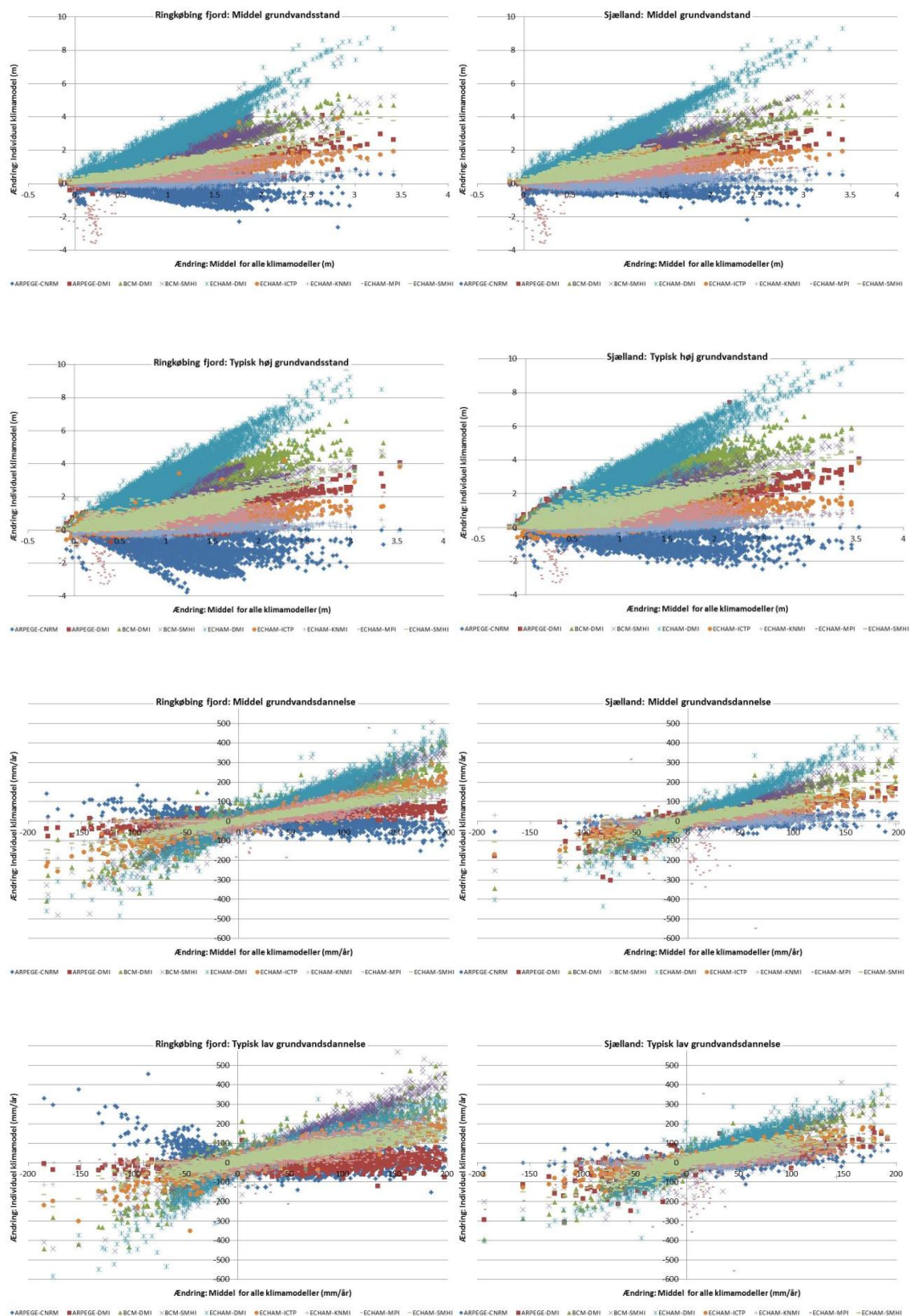
Figur 4.2 Resultater for Ringkøbing Fjord (venstre) og Sjælland (højre) af ændringer i mid-del grundvandstand (øverst, i meter), typisk høj grundvandsstand (næstøverst, i meter), middel grundvandsdannelse (næstnederst) og typisk lav grundvandsdannelse (nederst) i mm/år, 2021-2050 i forhold til 1961-1990.
