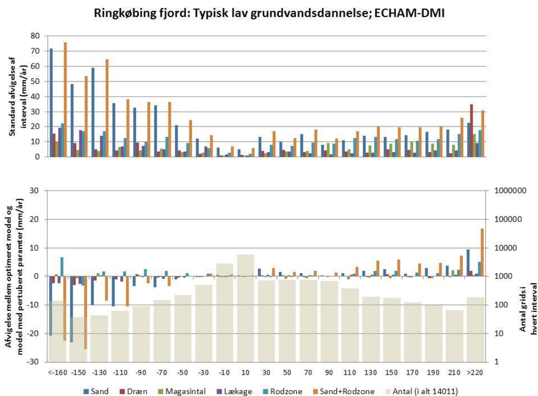
Fig. A2.12 Resultater for Ringkøbing fjord parameterusikkerheder: Ændring i typisk lav grundvandsdannelse i mm/år, 2021-2050 i forhold til 1961-1990.
