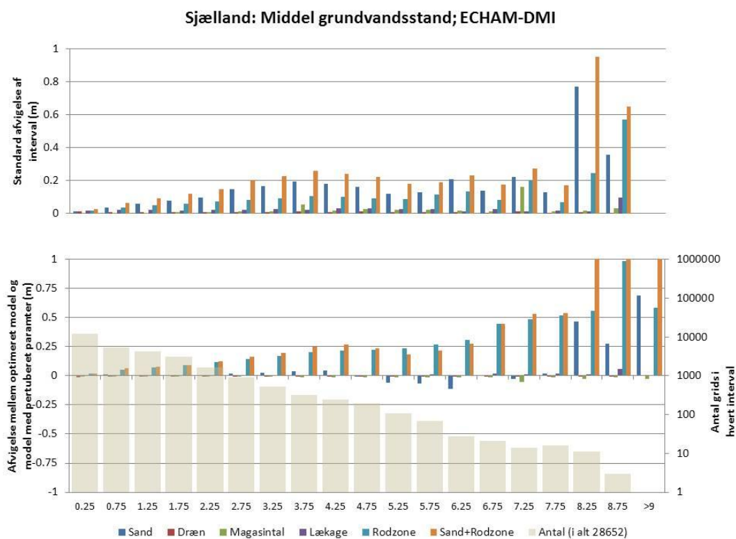
Fig. A2.13 Resultater for Sjælland parameterusikkerheder: Ændring i middel grundvandsstand i m, 2021-2050 i forhold til 1961-1990.
