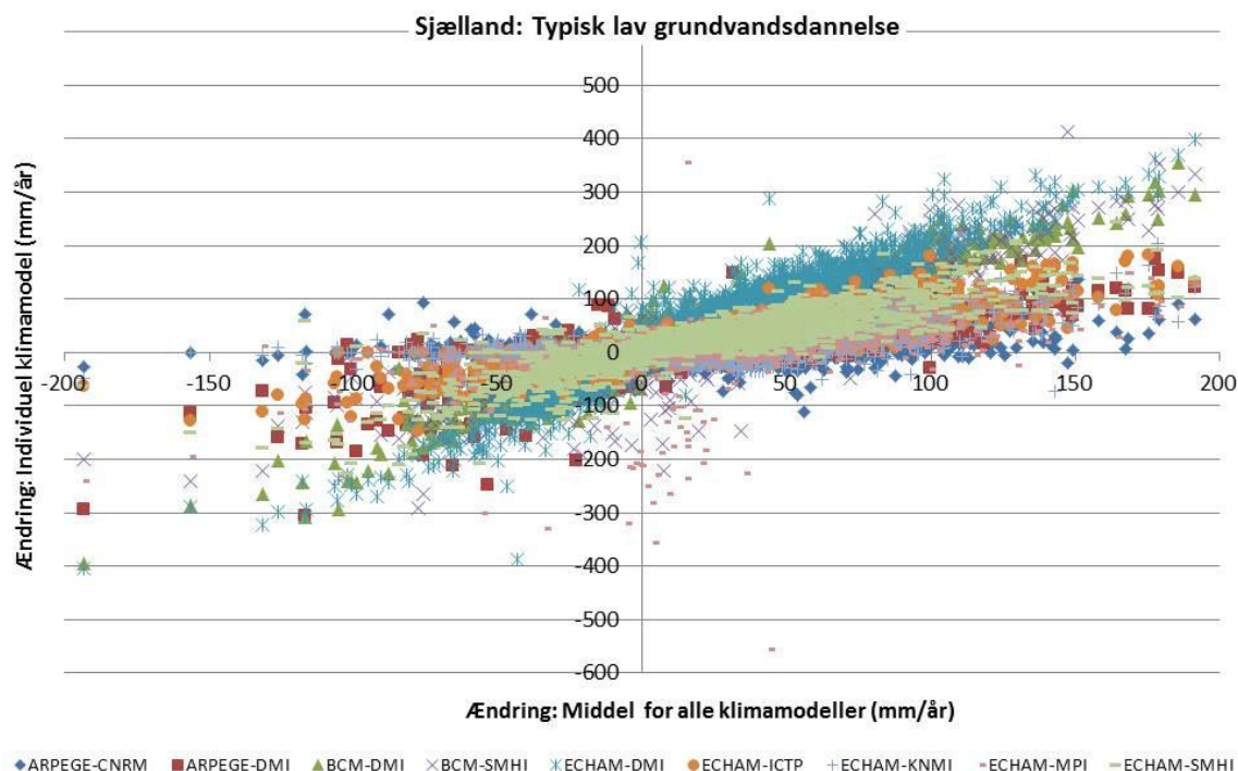
Fig. A2.8 Resultater for Sjælland inputusikkerheder: ændring i typisk lav grundvandsdannelse, i mm/år, 2021-2050 i forhold til 1961-1990.
