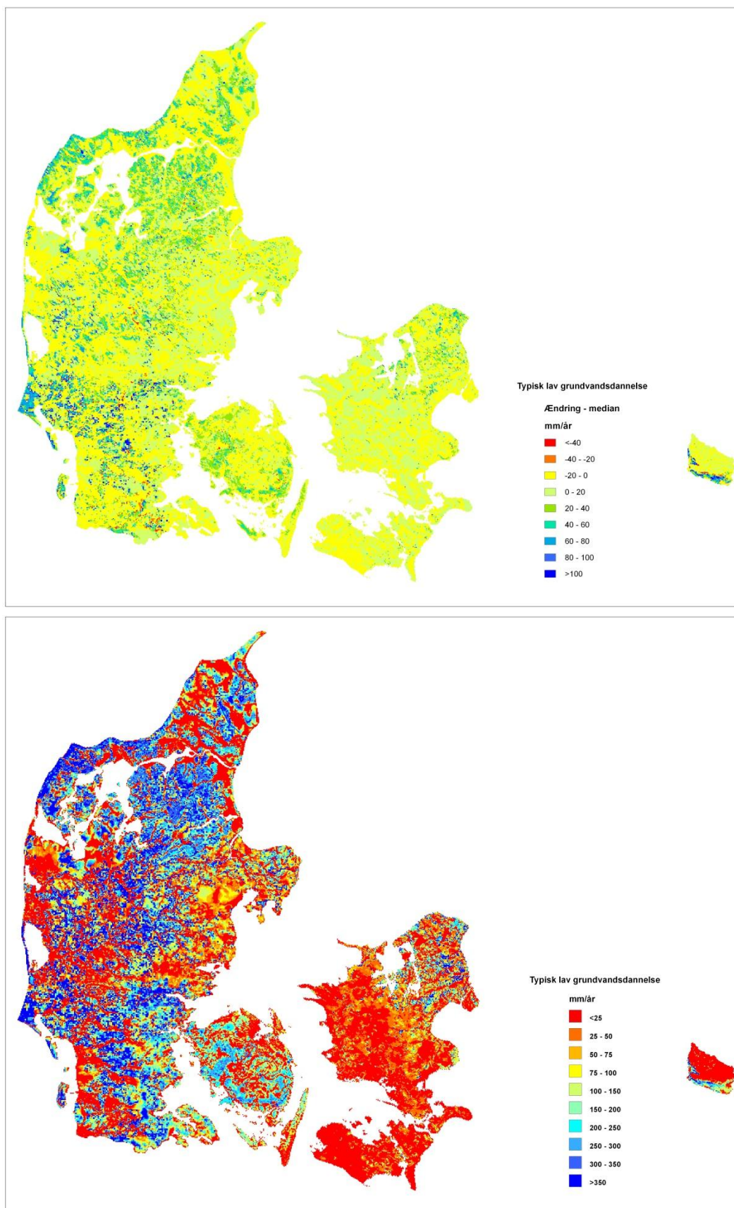
Figur 4.11 Ændring i typisk lav grundvandsdannelse "median klimamodel" 2021-2050 i forhold til 1961-1990. Nederst typisk lav grundvandsdannelse for kontrolperioden 1991-2010.
