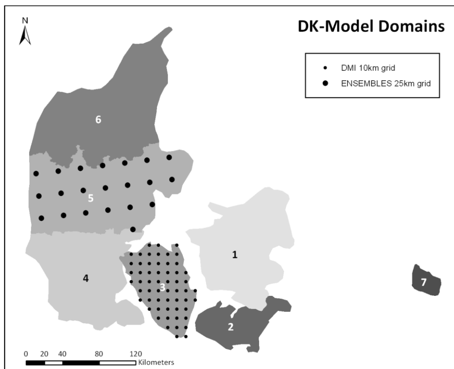
Figur 3.5 DK-model er opdelt i syv hydrologiske domæner, der anvender klimainput fra DMIs 10 km nedbørsgrid. Udfra 25 km klimamodelgrid (som vist for område 5) fra ENSEMBLES er der for hvert 10 km grid (som vist for område 3) interpoleret tidsserie-input fra de forskellige klimamodeller (Seaby et al., in prep).
