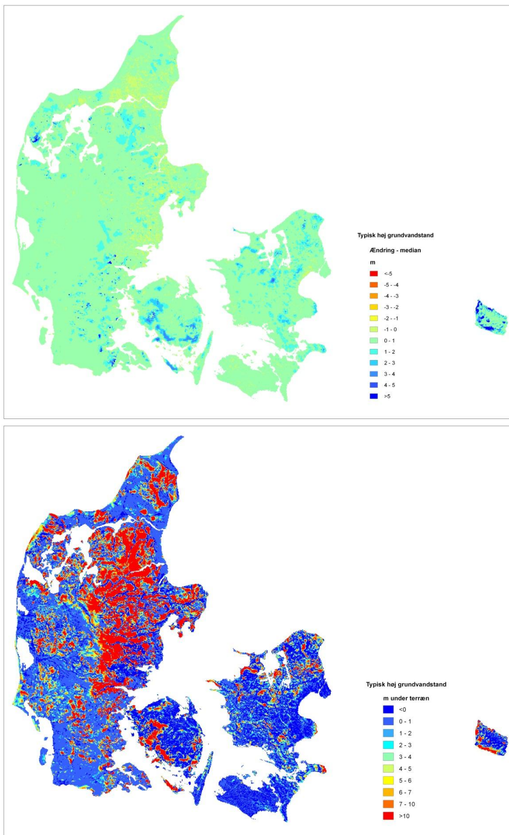
Figur 4.9 Ændring i typisk høj grundvandsstand for "median klimamodel" 2021-2050 i forhold til 1961-1990. Nederst dybde til typisk høj grundvandsspejl for kontrolperioden 1991-2010.
