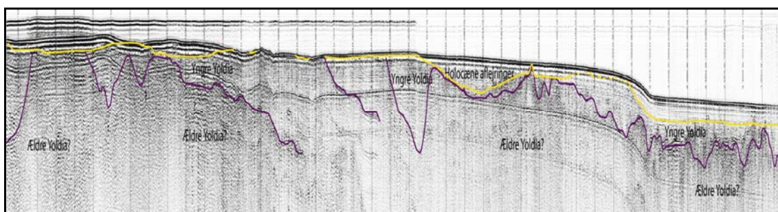
Figur 4.1 Seismisk profil linie Fred_1.
