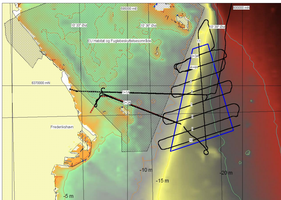
Figur 2. Seismik undersøgelser i havvindmøllepark ved Frederikshavn.
