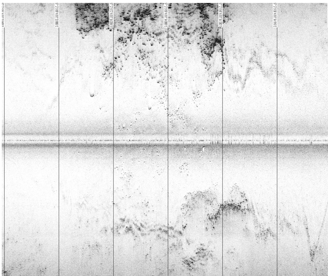
Figur 6.6 Udsnit af Side scan sonar data, Fred_1, med stenbestrøning.
