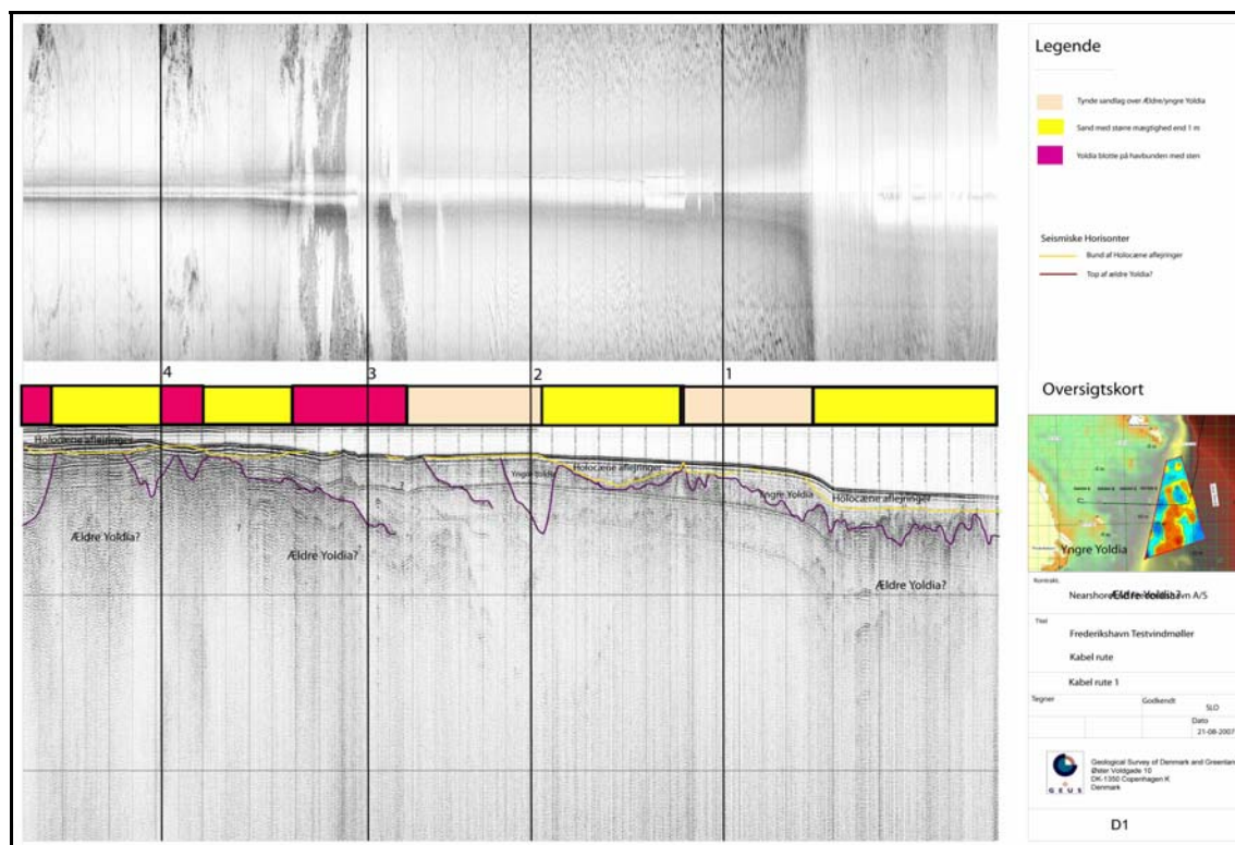
Figur 6.2 Nordlige kabel rute, sammenstillede data (Bilag D1).
