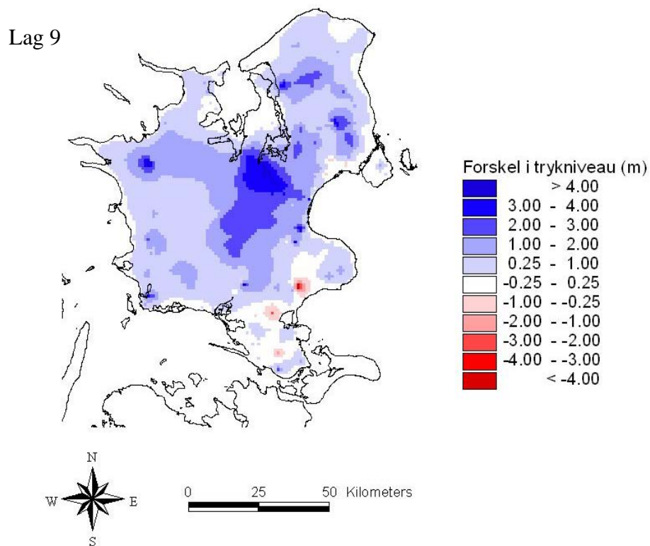
Figur 12 Forskel i trykniveau-udvikling 1989-2001 for hhv. simulering med aktuelle indvindingsrater og indvindingsrater fastholdt til 1989-niveau.
