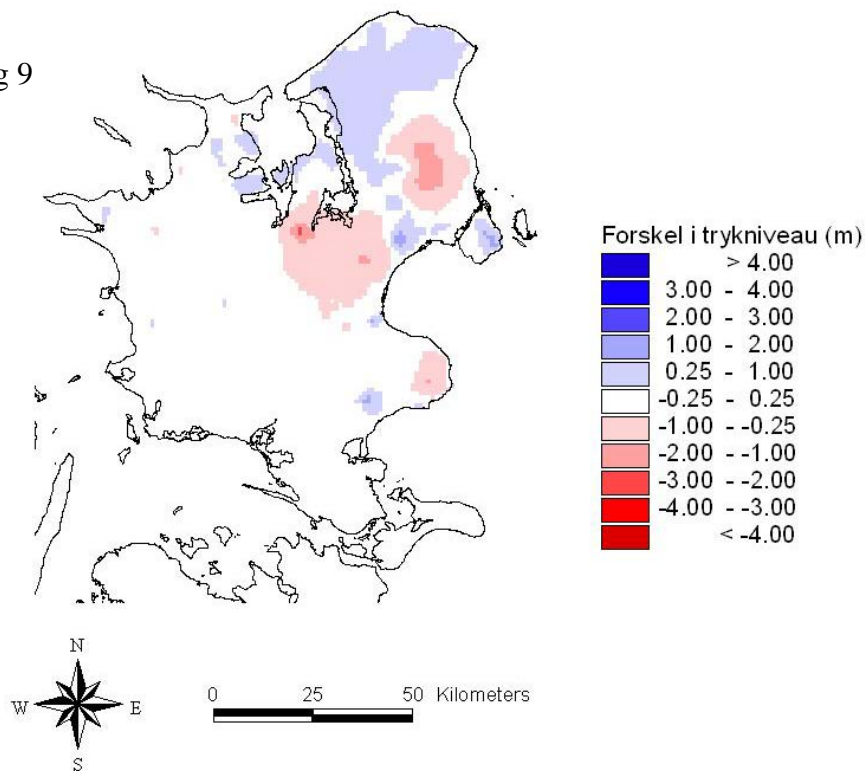
Figur 11 Forskæl mellem trykniveauet 2001 og 1989 for hhv. beregningslag 3 og 9 (indvinding fastholdt til 1989-niveau).
