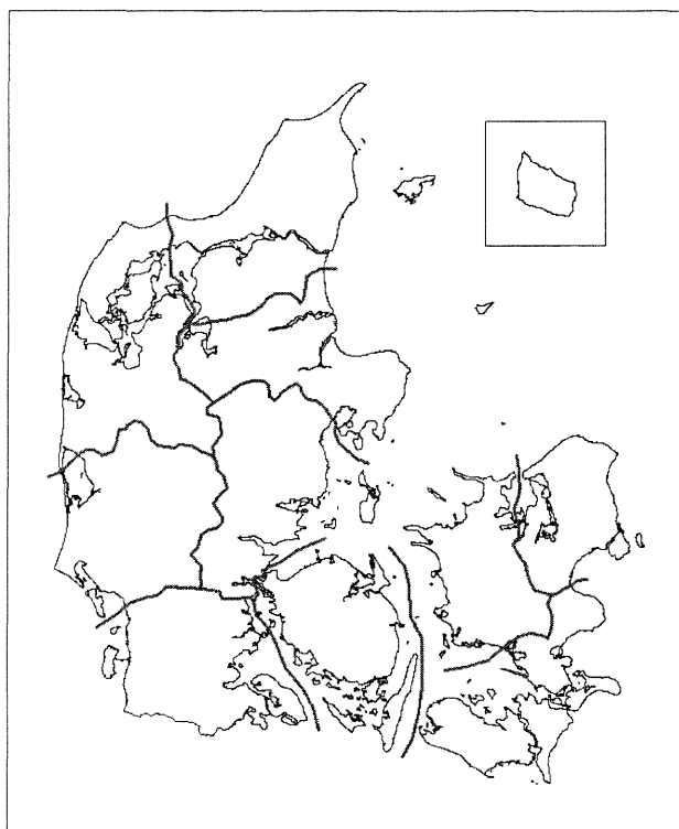
Figur 3.1 Opdeling af DK-model på 11 regionale delmodeller
