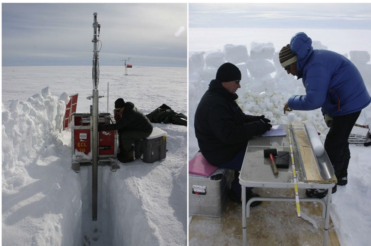
Figur 1: Boring af firnkerner med Eclipse2-systemet (venstre) samt måling af firnens densitet (højre).
